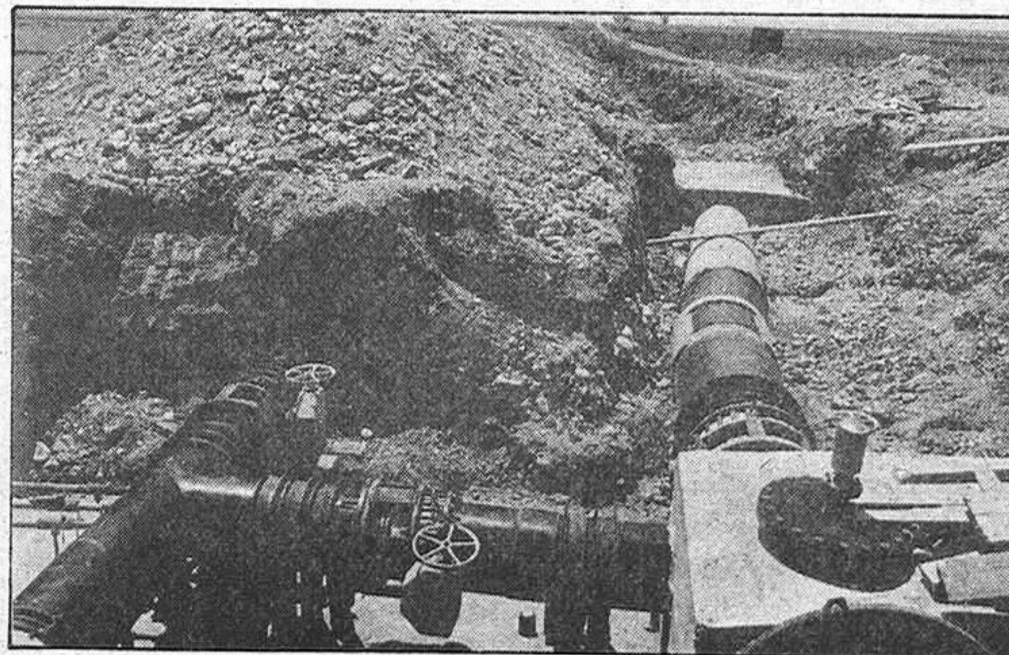
Obras del desdoblamiento Marchamalo-Alcalá de Henares.
