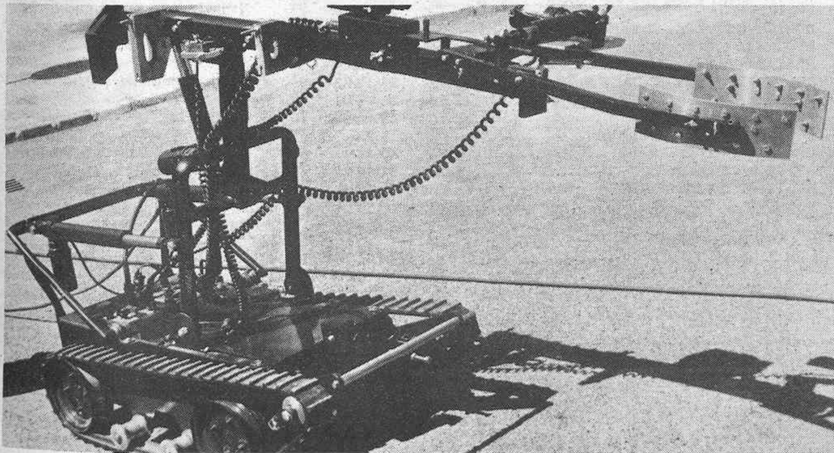
El montaje en oruga le permite acceder a terrenos difíciles y diversos.
