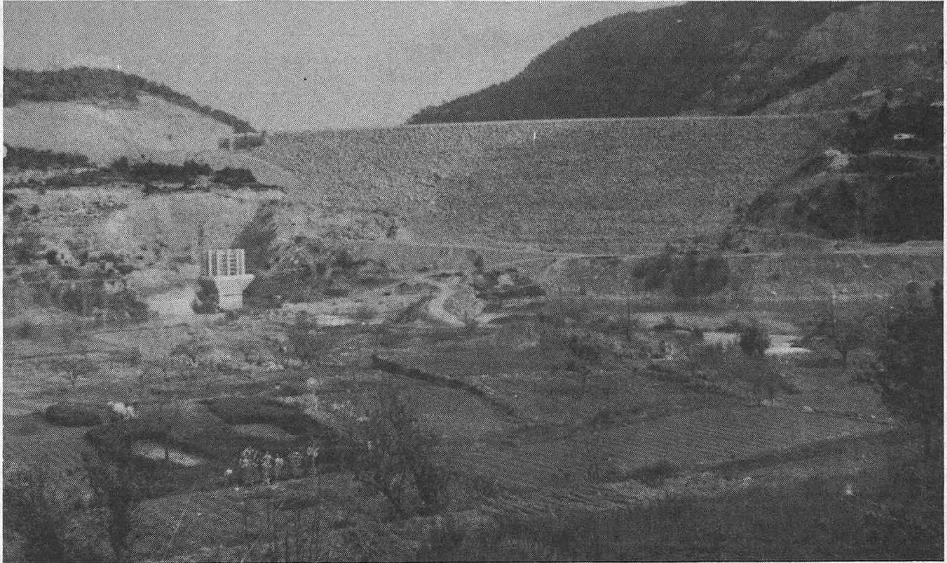
Presa de Arenós, de materiales sueltos, durante el período de construcción
