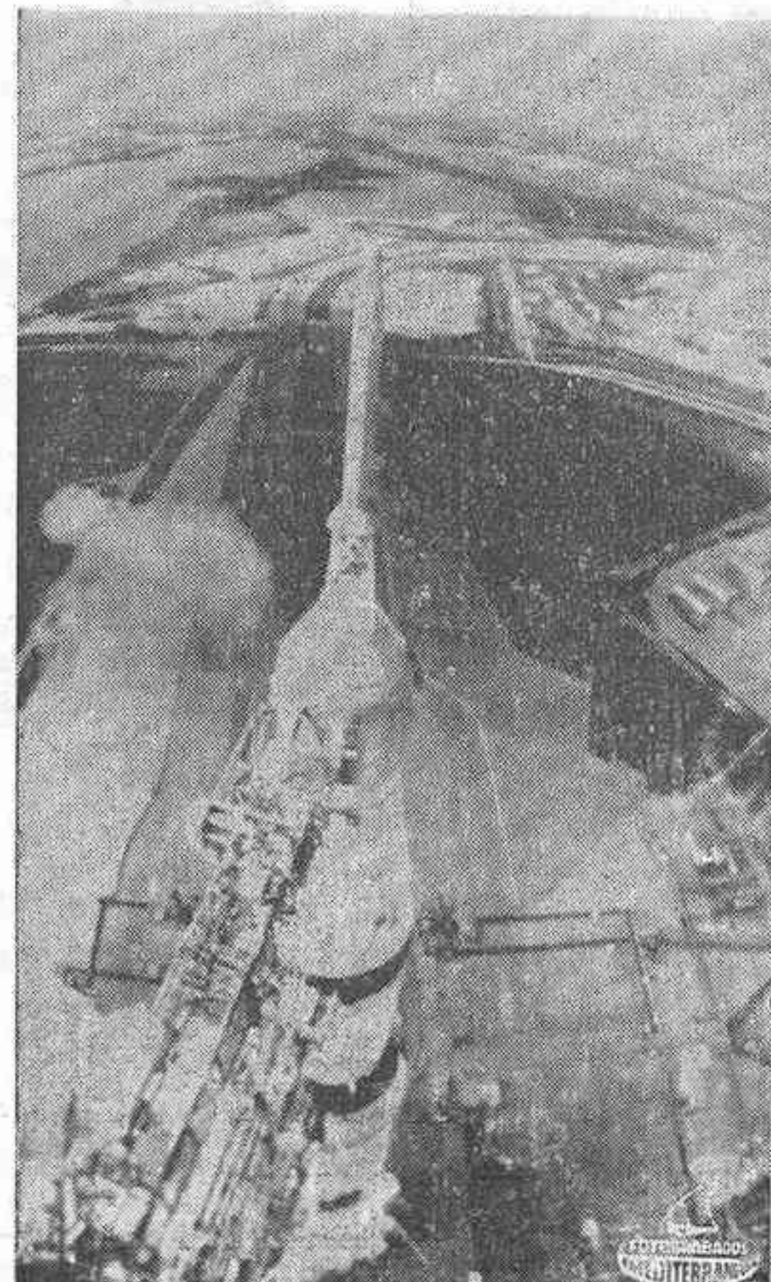
CABO KENNEDY. — El Apolo XV que el próximo día 26 saldrá para la Luna ha hecho sus pruebas de funcionamiento en el gigantesco cohete Saturno. En la foto, tomada por una máquina automática, se ve cómo el vapor de oxígeno sale hacia la atmósfera en un momento de las pruebas realizadas el pasado día 13. — (Telefoto CIFRA)
