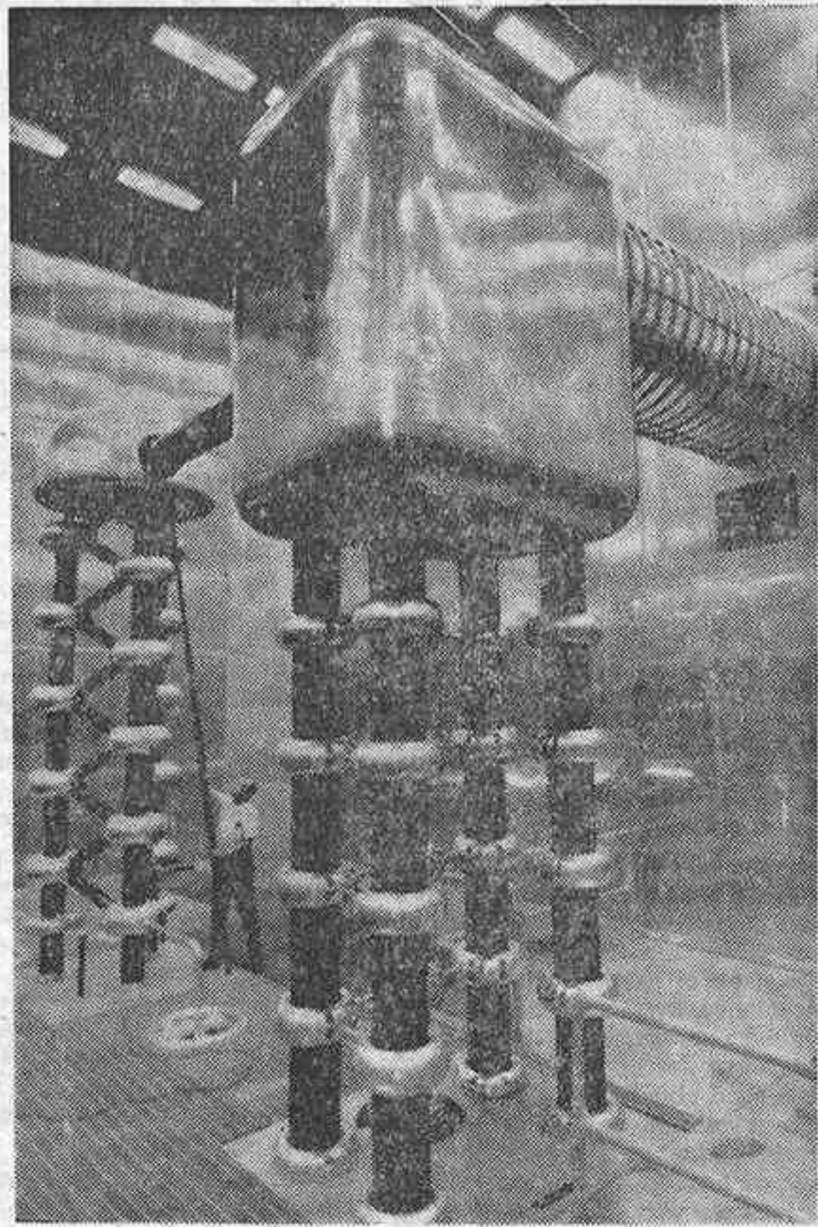
Sistema de generación de un nuevo acelerador de protones de un coste de 56 millones de dólares, actualmente en construcción en las Instalaciones para Estudio de la Física sobre los Mesones de la Comisión de Energía, en Los Alamos (Nuevo México). Podrá desintegrar las células cancerosas en explosiones nucleares en miniatura.—(Foto Pyresa)
