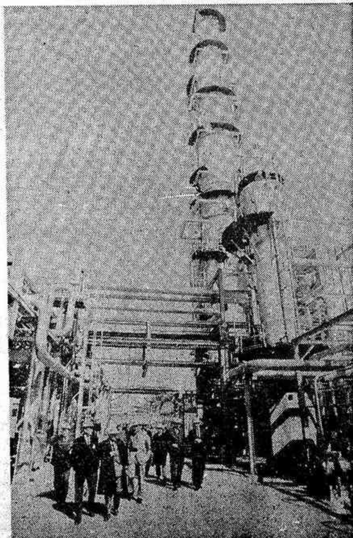
La capacidad de refino actual de la planta de Castellón comprende un diez por ciento del total nacional. La ampliación incrementará notablemente este índice
