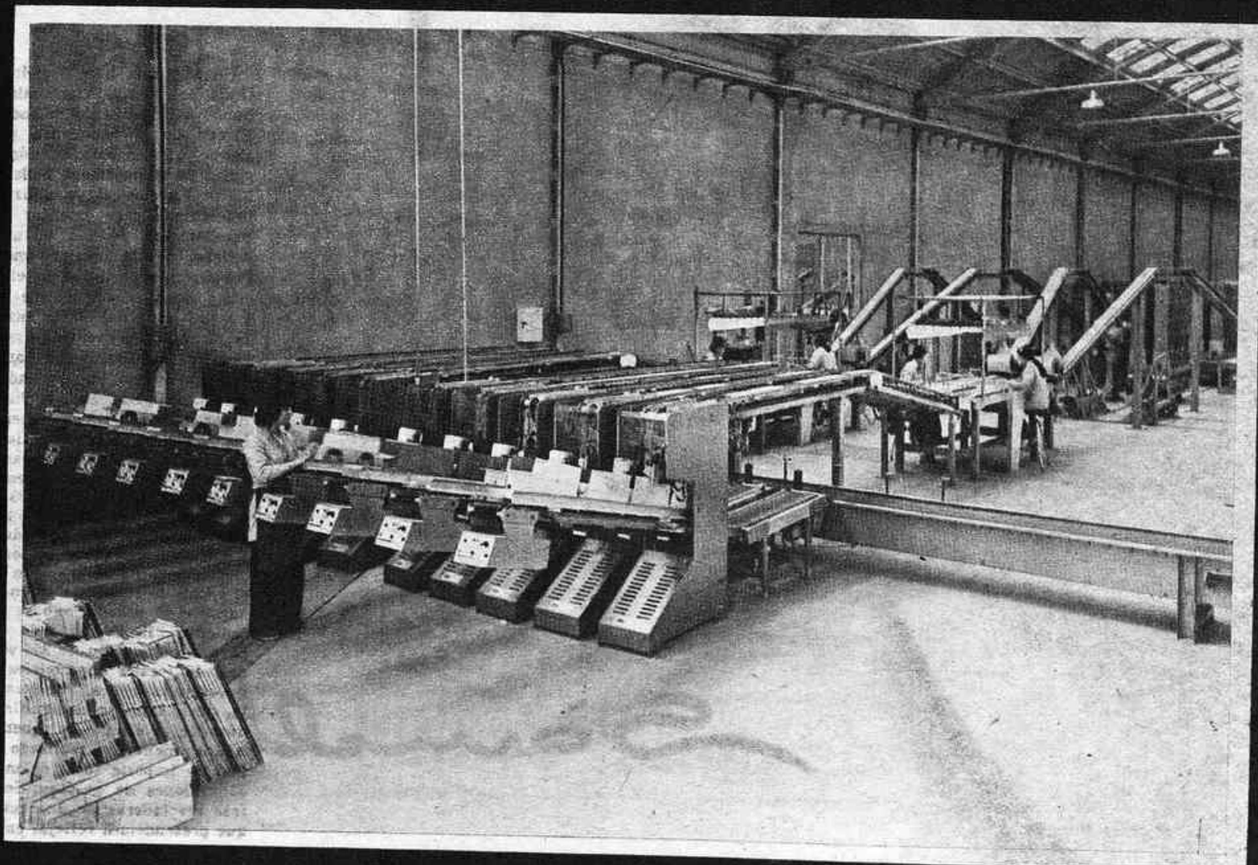
LINEA DE SELECCION Y ENVASADO AUTOMATICO
