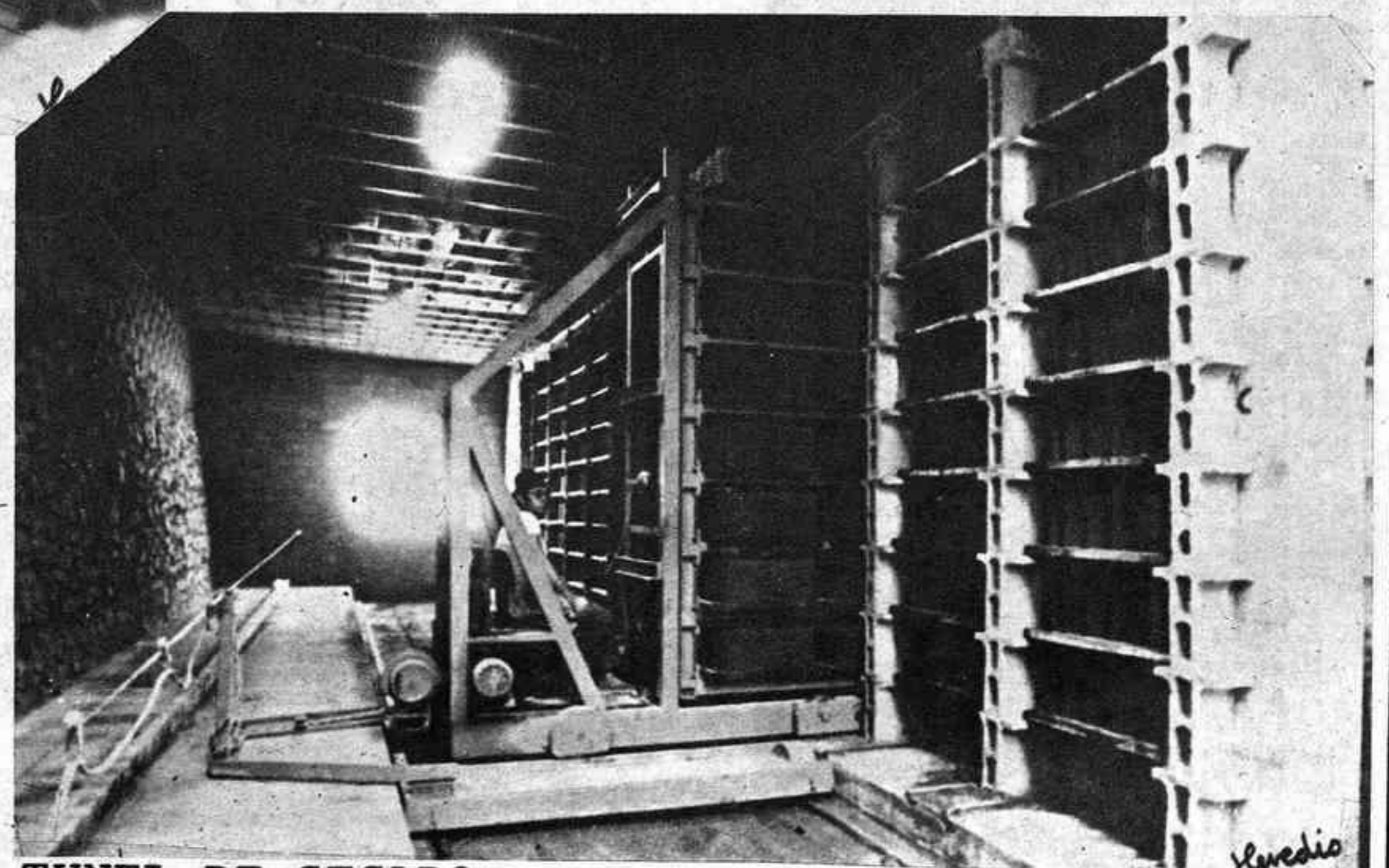
TUNEL DE SECADO
