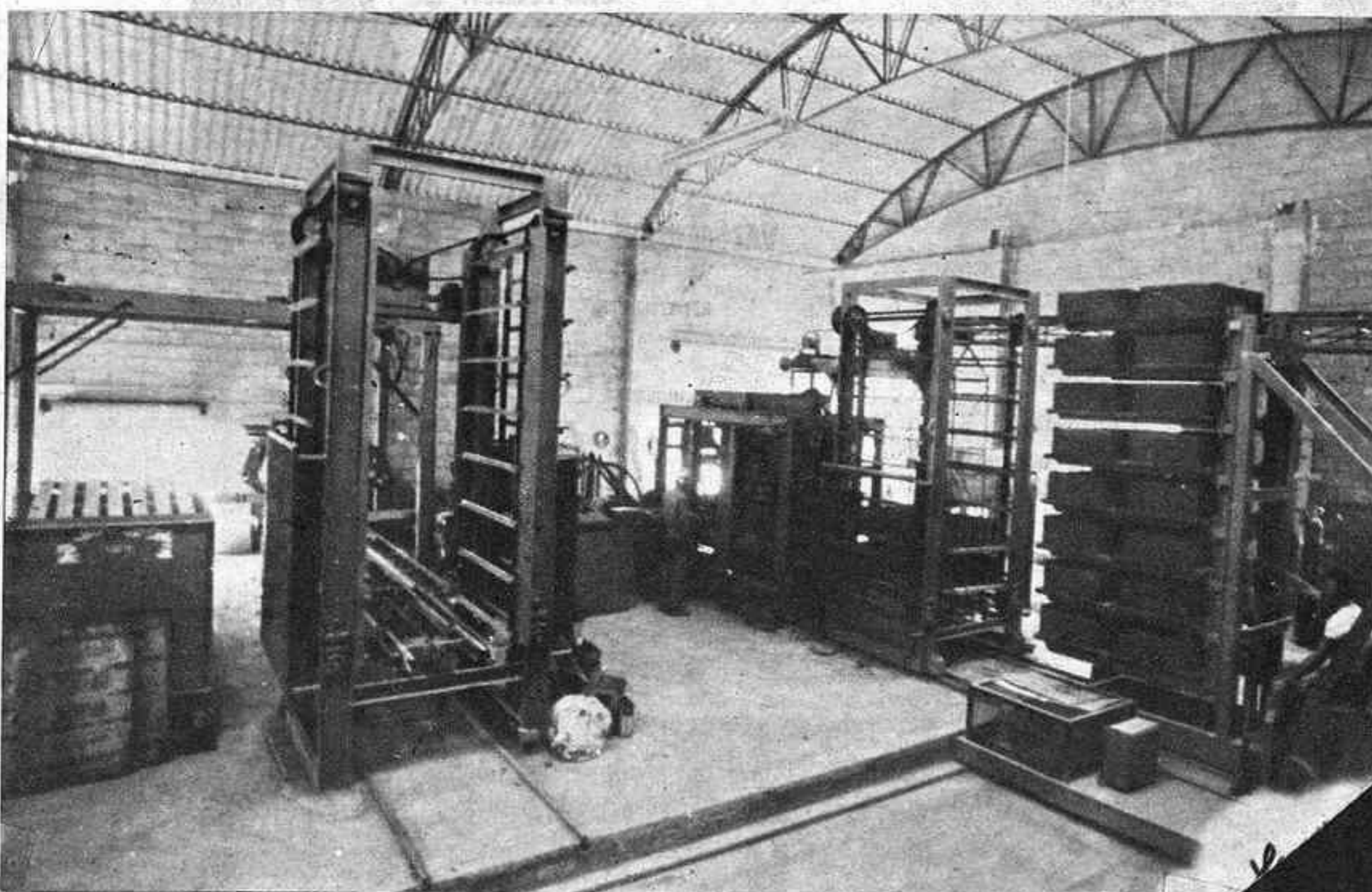
INSTALACION AUTOMATICA PARA FABRICACION DE VIGUETAS
