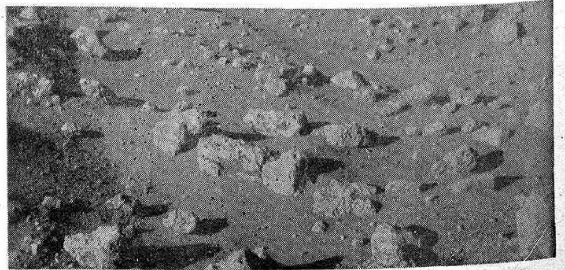
PASADENA (California).—La fotografía muestra el lugar cerca del cual ha aterrizado el «Vikingo II». Posiblemente sea de aquí de donde se toman las muestras de tierra para analizar. La mayoría de las rocas de esta zona tienen una apariencia porosa. Este aspecto en la Tierra lo habrían adquirido a través de un proceso volcánico o del impacto de los meteoritos. Un volcán próximo al lugar pudiera ser la causa de estas rocas.—(Telefoto Cifra Gráfica)
