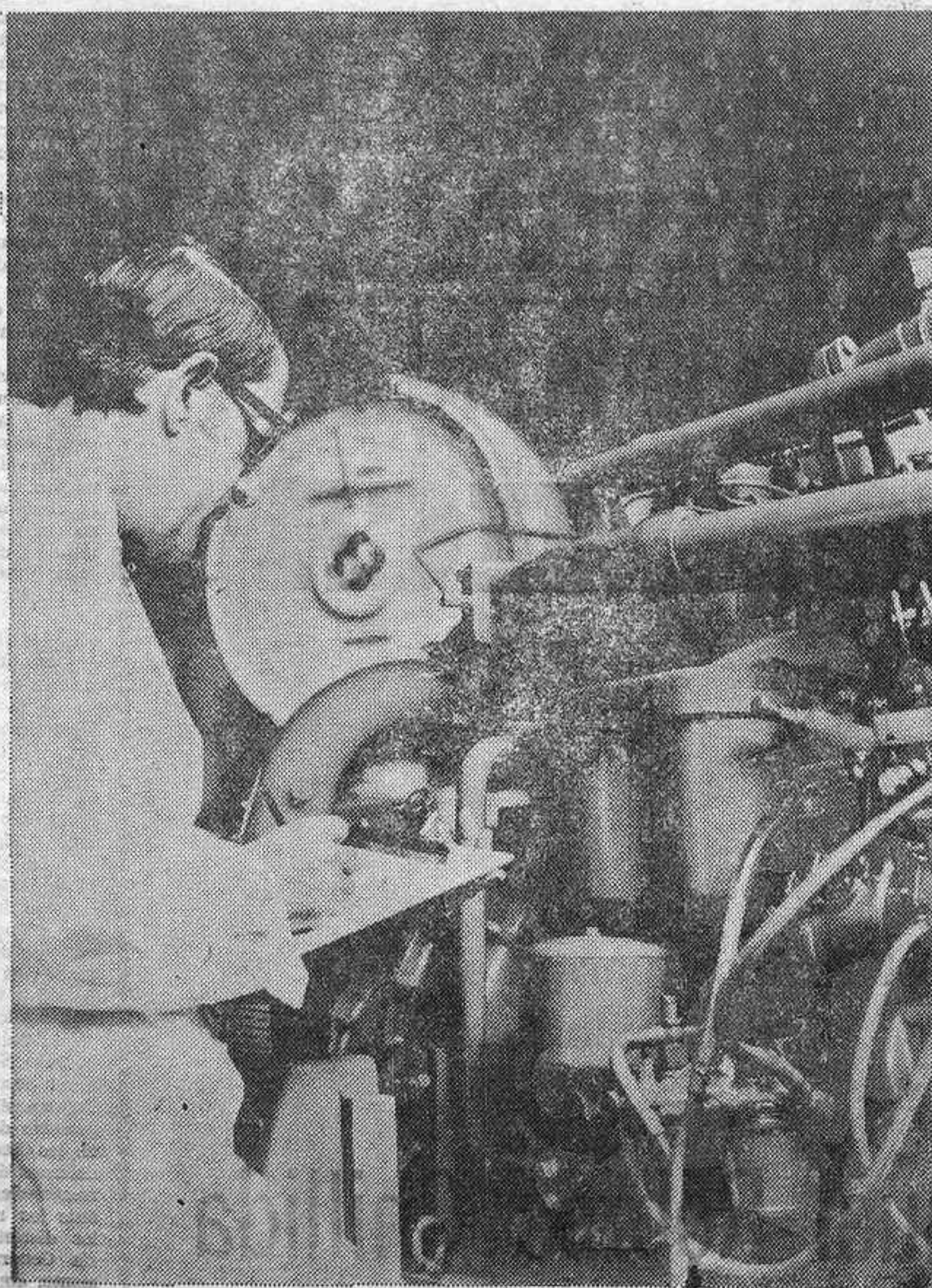
Motor experimental M3BB36VSU. Comprobación de potencias a diversas revoluciones.
