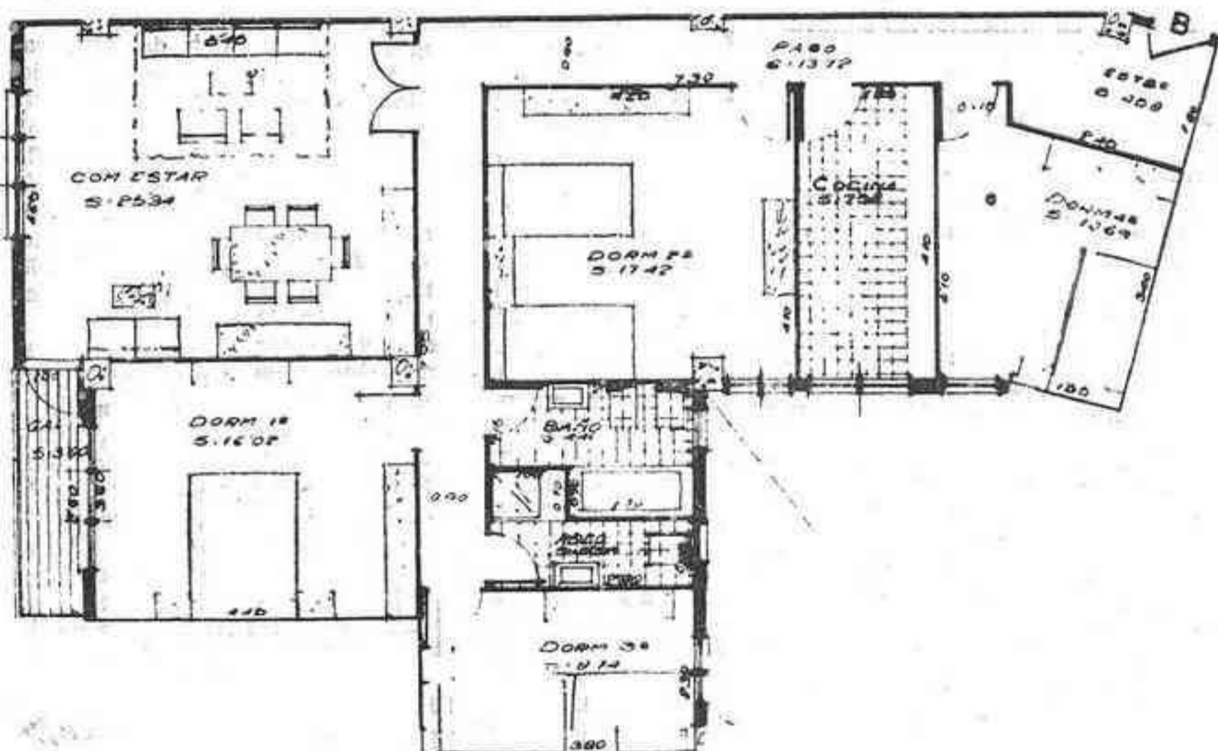
VIVIENDA TIPO -B-
