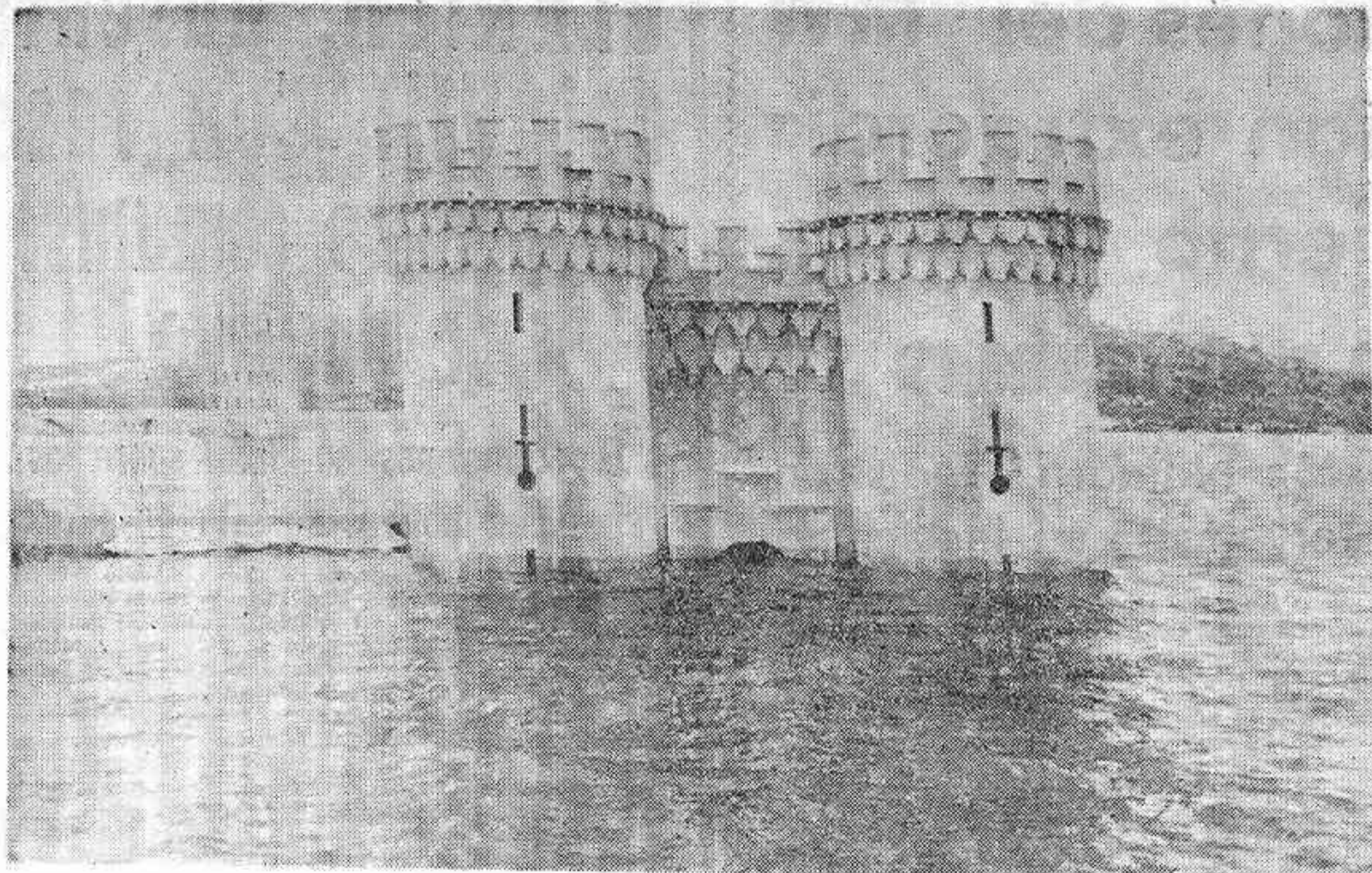
MADRID.- El ministro de Obras Públicas, Fernández de la Mora, acompañado por el ministro inglés de Transportes, John Peyton, inauguró la nueva presa de Manzanares el Real, ampliación de la antigua presa construida por Hidráulica Santillana, y que surtirá de agua a Madrid. En la foto, el agua cubriendo parte de las antiguas torres de la presa primitiva. (Telefoto Cifra Gráfica).
