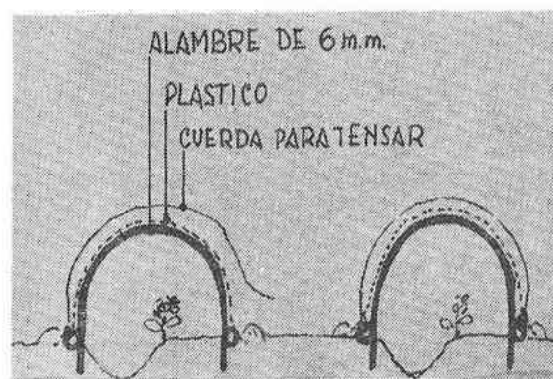
La "cuerda para tensar" puede atarse en los bucles y éstos, formados con el alambre de 6 mm, impiden que unos se claven en tierra más que otros.
