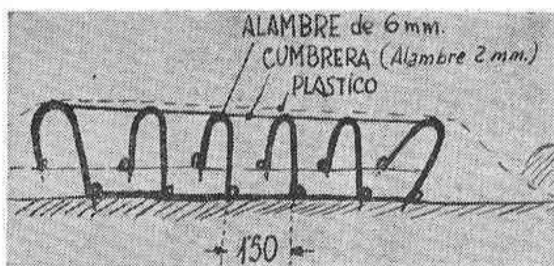
Los alambres de 6 mm se ponen a 150 mts. de distancia y los finales se inclinan para que hagan de tensores del plástico.
