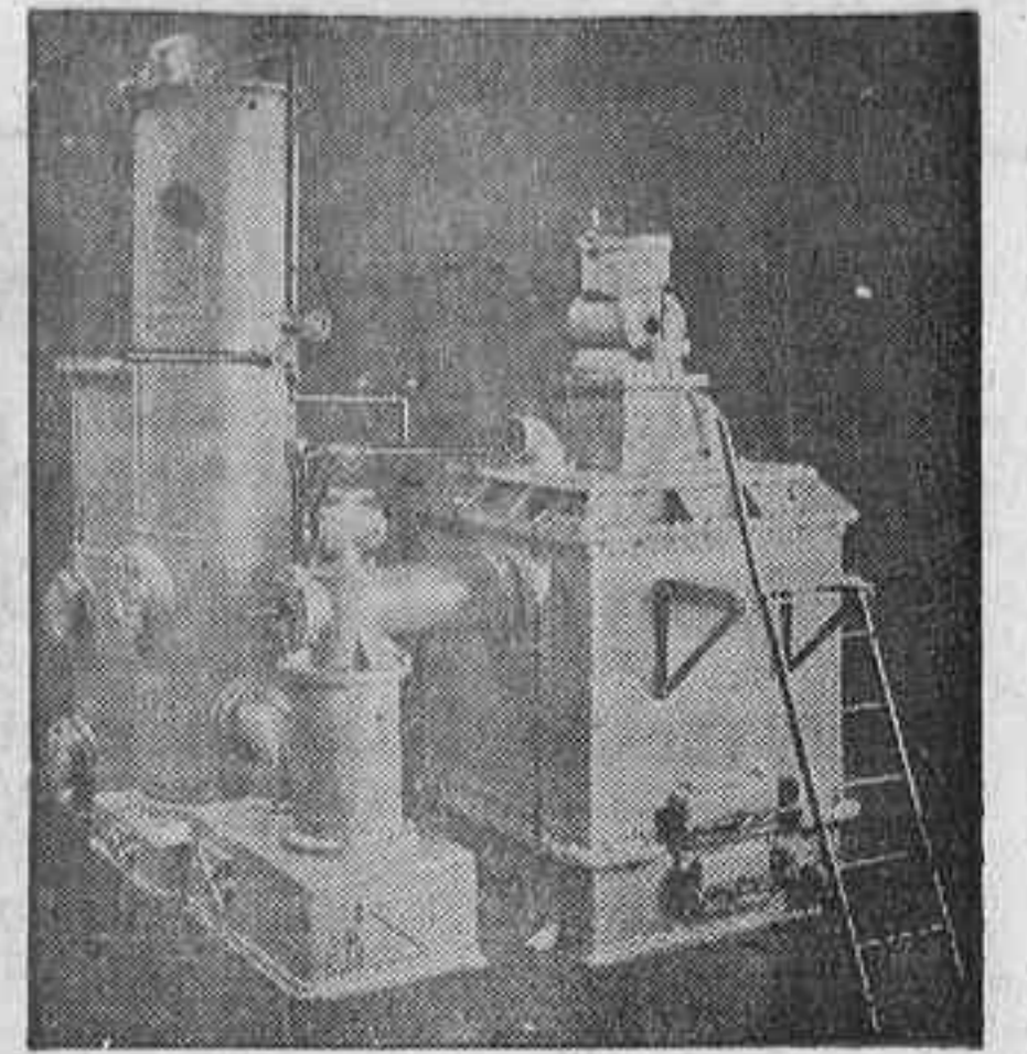
Gasógeno sencillo
