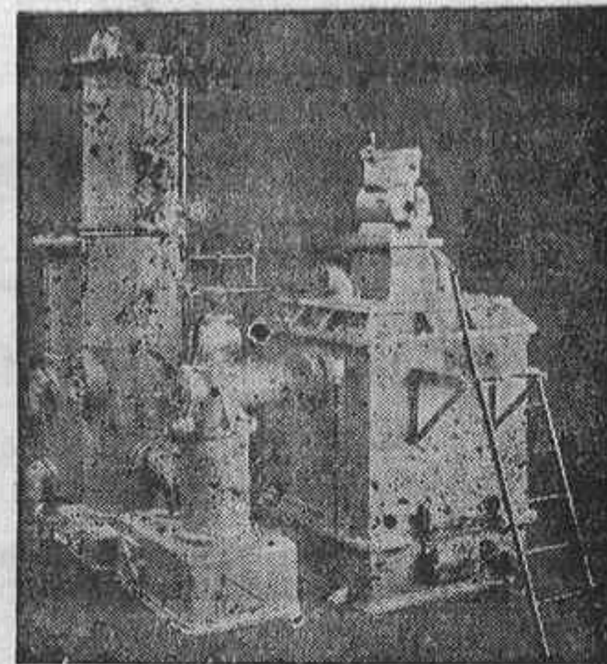
Gasógeno sencillo
