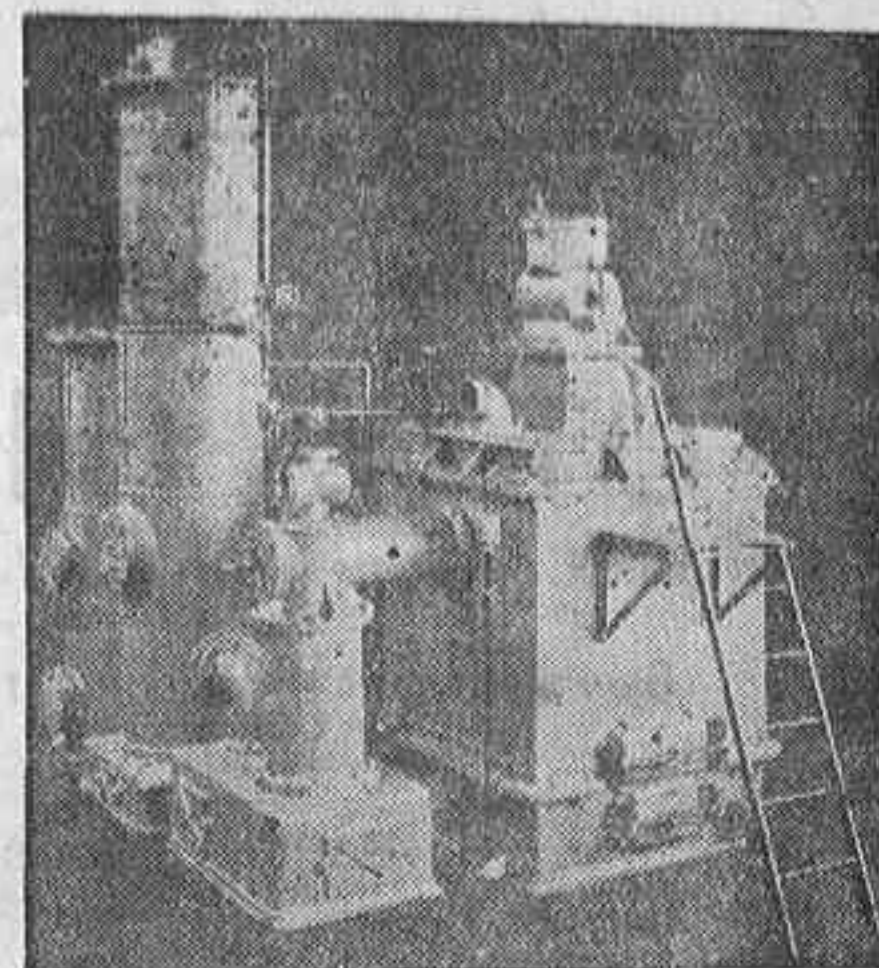
Gasógeno sencillo
