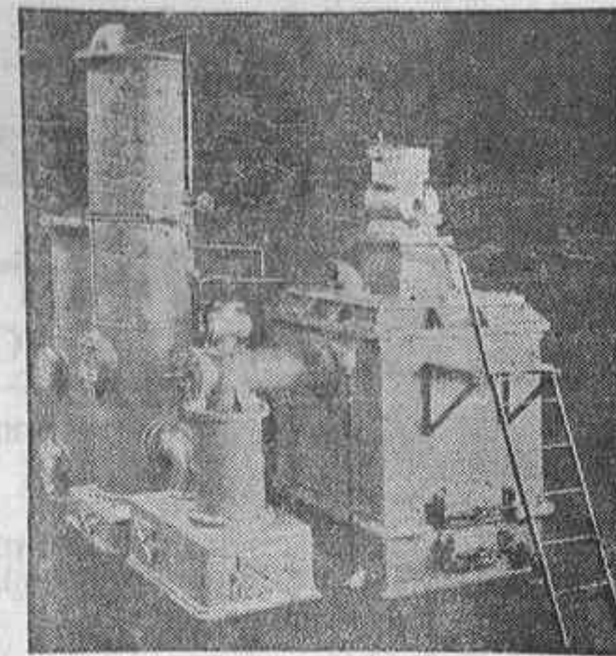
Gasógeno sencillo
