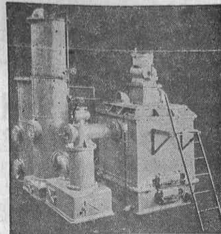
Gasógeno sencillo
