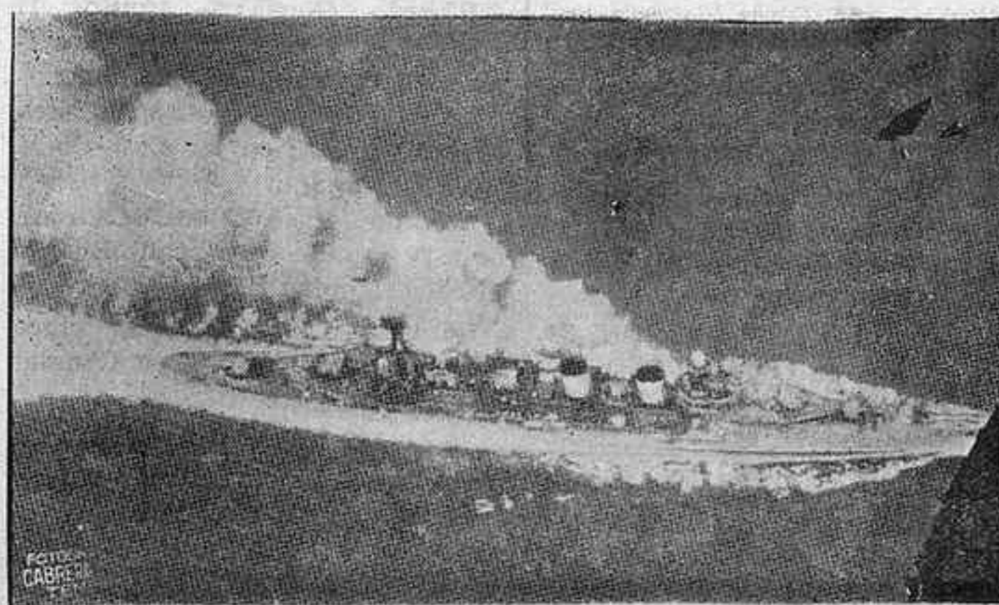
Crucero "Almirante Cervera.—Desplazamiento, 7.975 toneladas; velocidad, 33 millas; 8 piezas de 152,5 m/m, 4 de 101,6 m/m anti-aéreos, 2 de 47,5 m/m y 12 tubos de lanzar torpedos. Manda este buque el capitán de Navío don Francisco Basquerchi
