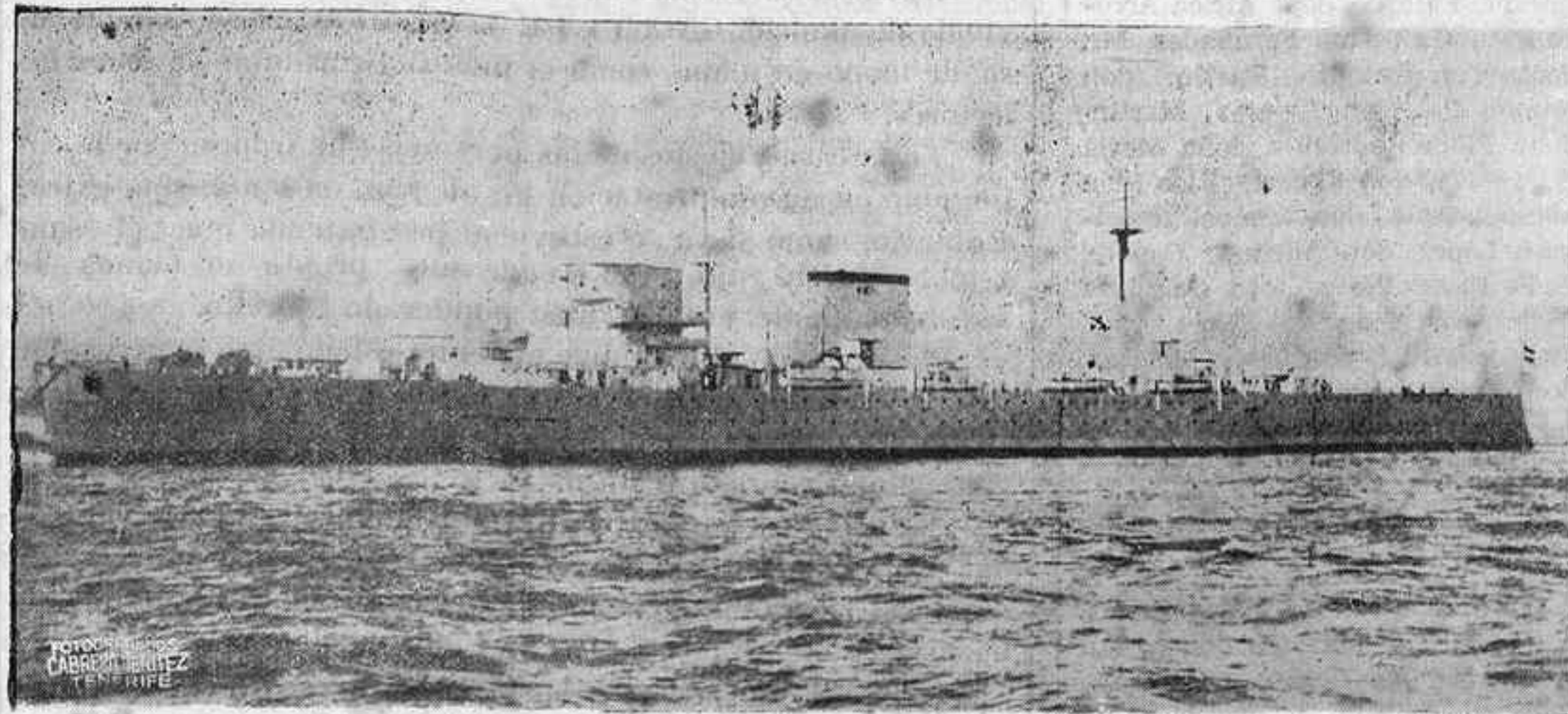
EL "CHULO" DEL MEDITERRANEO.—Crucero "Canarias": Las características de este buque son las siguientes: Desplazamiento, 10.000 toneladas; velocidad, 34 millas; 8 piezas de grueso calibre de 203,5 m/m, 6 de 120,5 m/m, 4 de 120,45 m/m anti-aéreos y 12 tubos de lanzar torpedos. Lleva también dos hidroaviones. En este buque arboló su insignia el jefe de la flota nacionalista, capitán de Navío don Francisco Moreno
