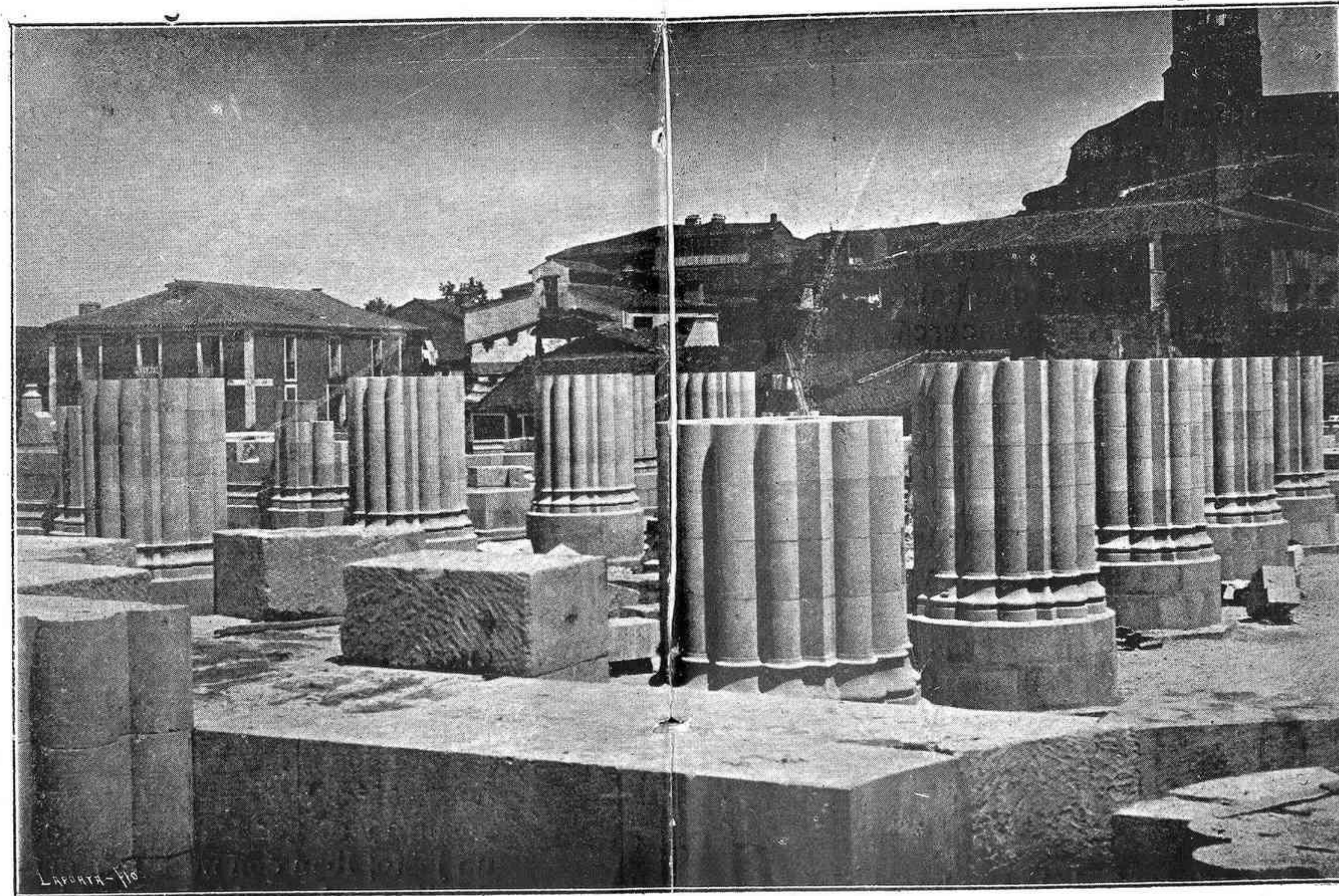
BASÍLICA EN CONSTRUCCIÓN DE SANTA TERESA DE JESÚS EN ALBA DE TORMES.—Estado de las obras en 20 de Mayo de 1904
