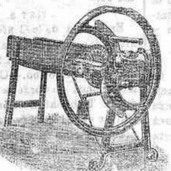
Cortaforrajes Columbus
