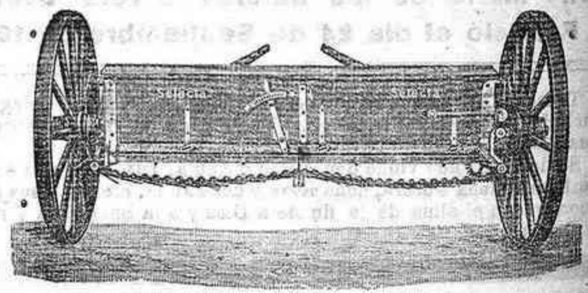
Distribuidora Westfalia
