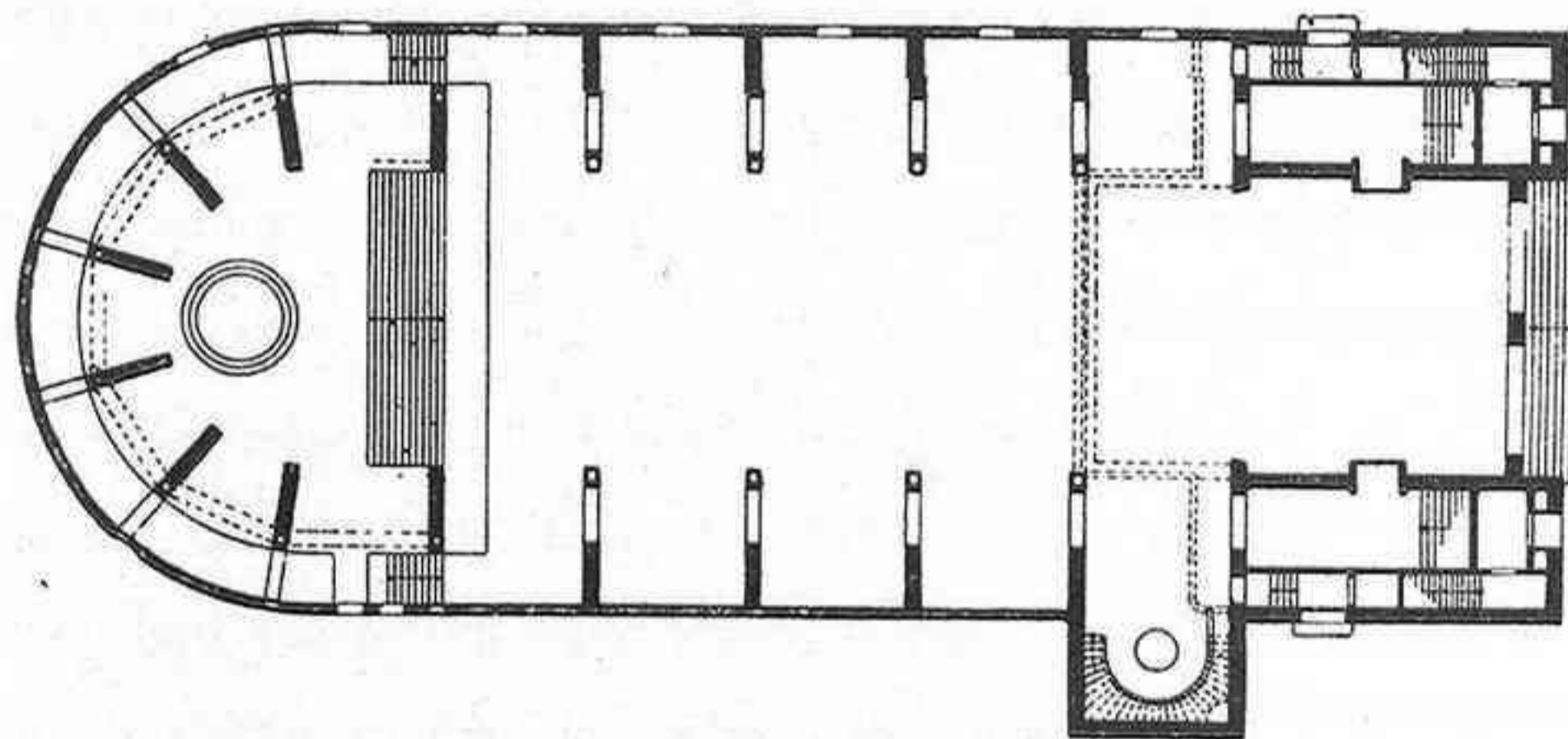
Iglesia de San José en Hindenburg. Planta.
