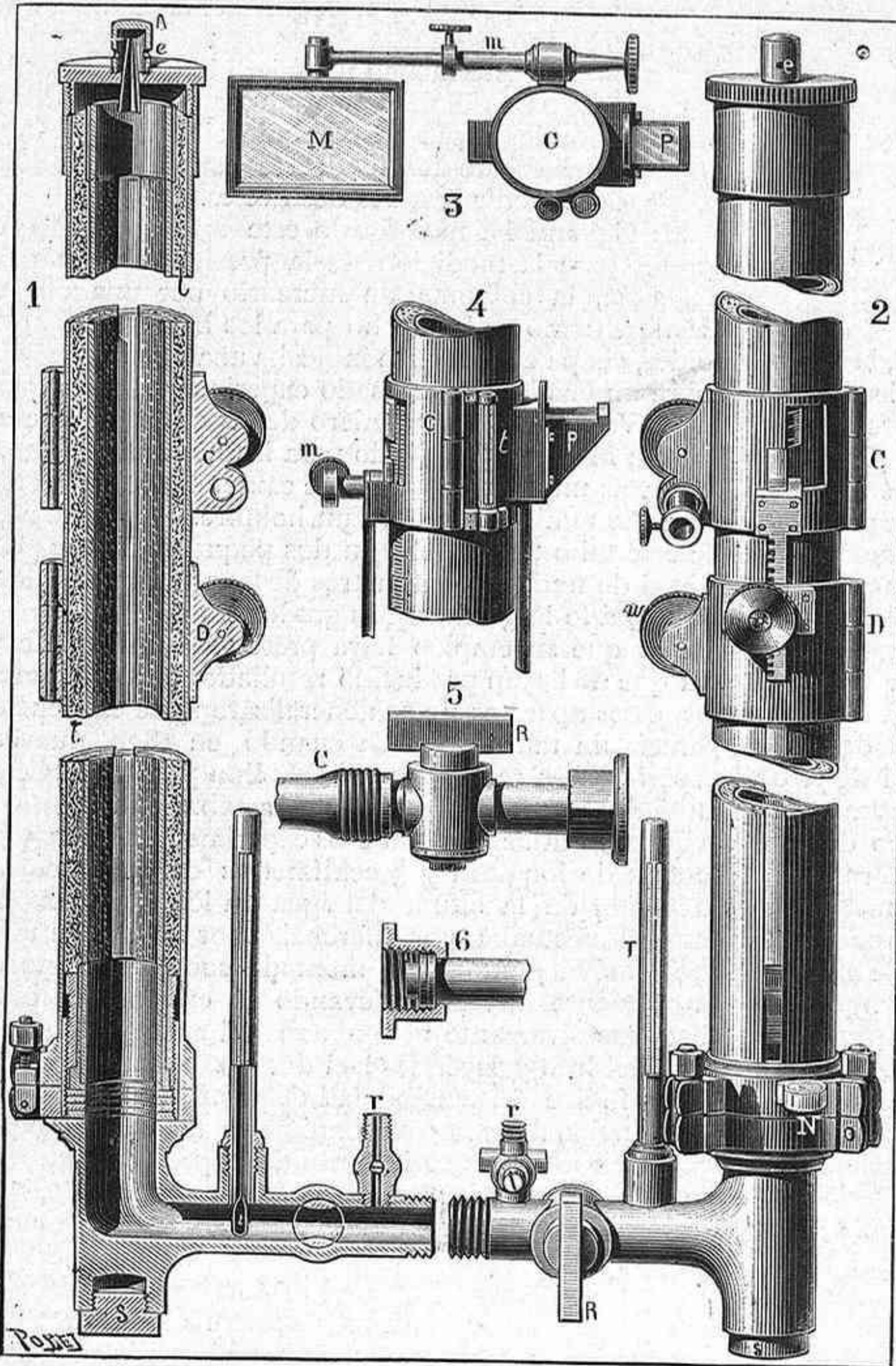
Fig. 1. - Nivel de agua de largo alcance. - Dibujos de detalle. - 1, Sección vertical de un tubo. - 2, Elevación de un tubo. - 3, Cilindro de puntería con el espejo, visto de frente. - 4, Cilindro de puntería visto de perfil. - 5, Enlace con el tubo de comunicación. - 6, Sección de un enlace de comunicación.
