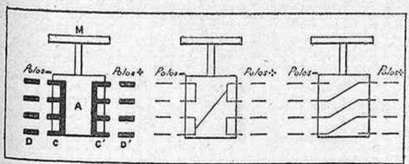
Fig. 3. Aparato para acoplar los acumuladores
