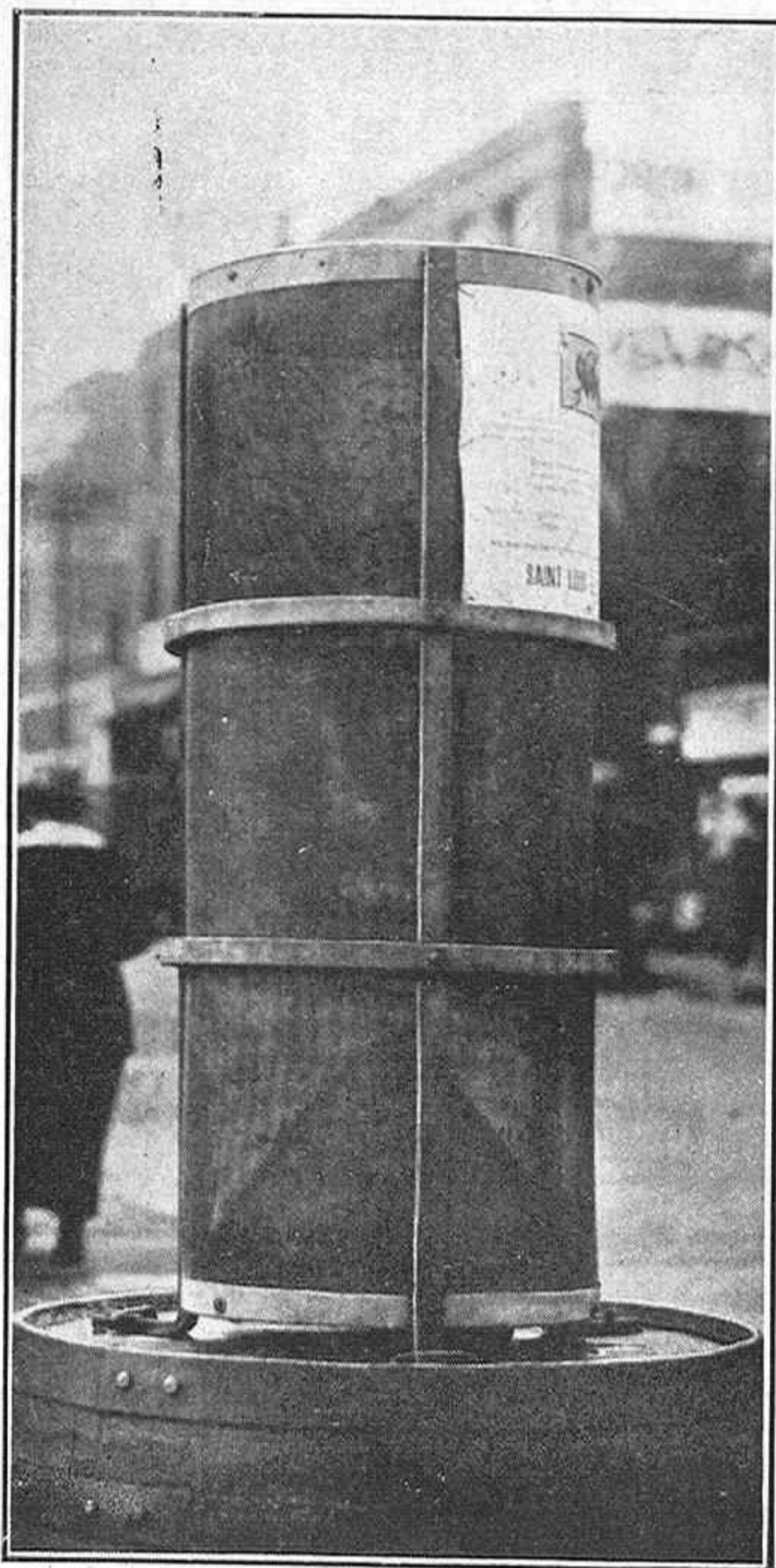
Ingenioso aparato caza-moscas, que ha sido instalado en las calles de San Luis (Estados Unidos), para contribuir de un modo rápido y eficaz á la extinción de la molesta y pernicioso plaga
