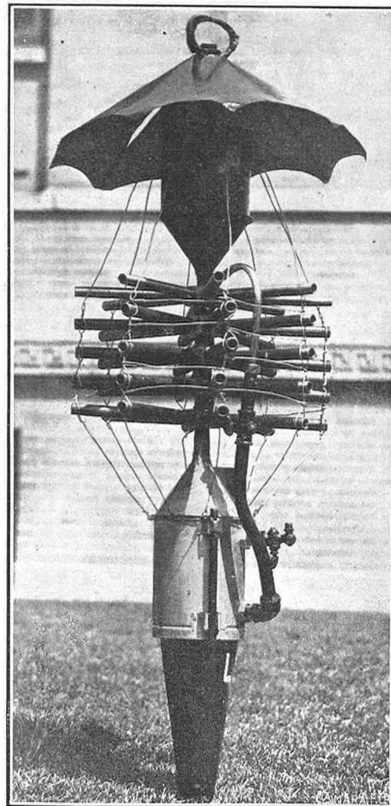
Nuevo aparato que al ser lanzado por una aeronave clábase en el suelo é irradia una luz vivísima que facilita los reconocimientos nocturnos, yendo provisto de cañoncitos que disparan en todas direcciones
