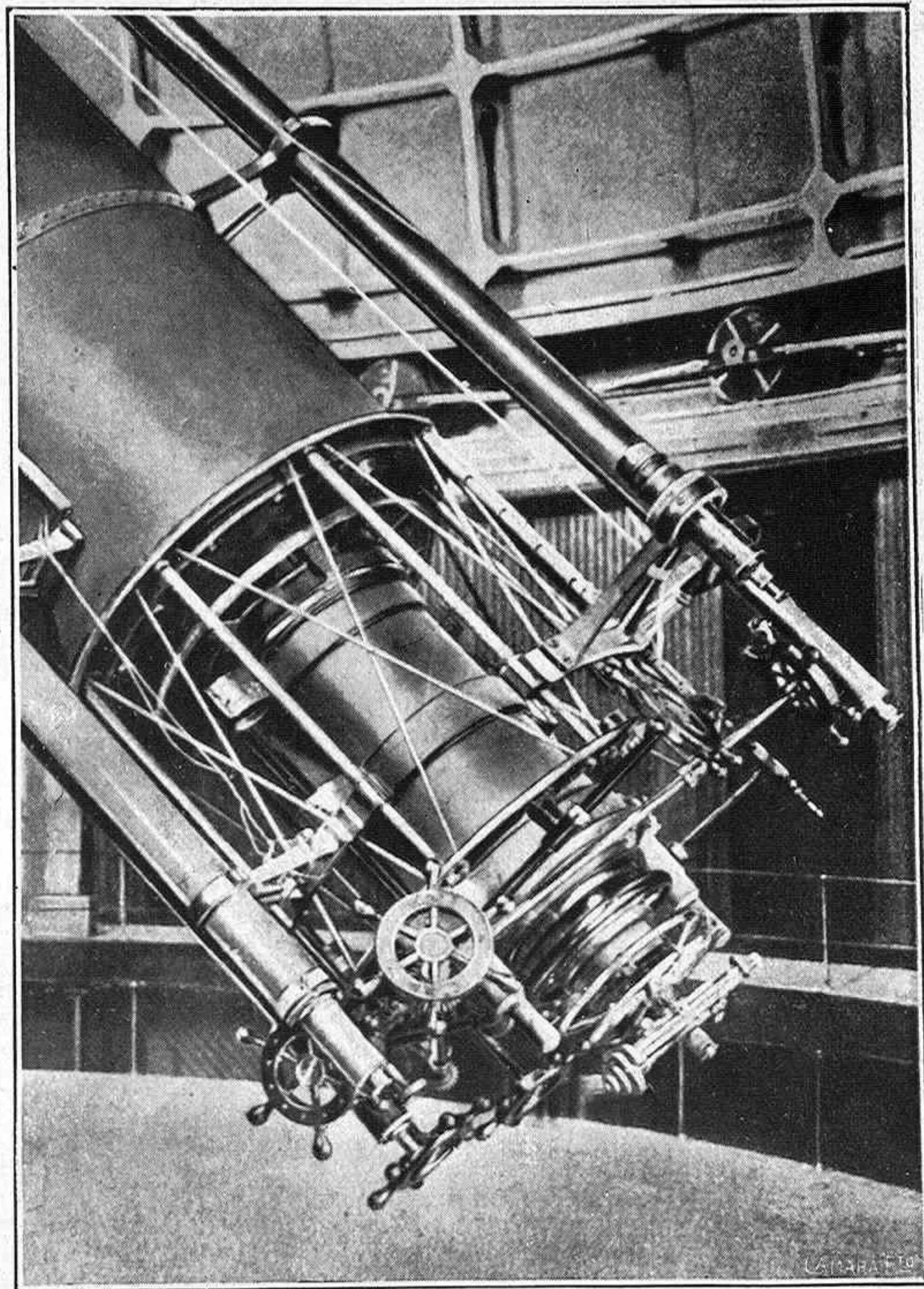
Ocular del gran refractor del Observatorio de Lick
