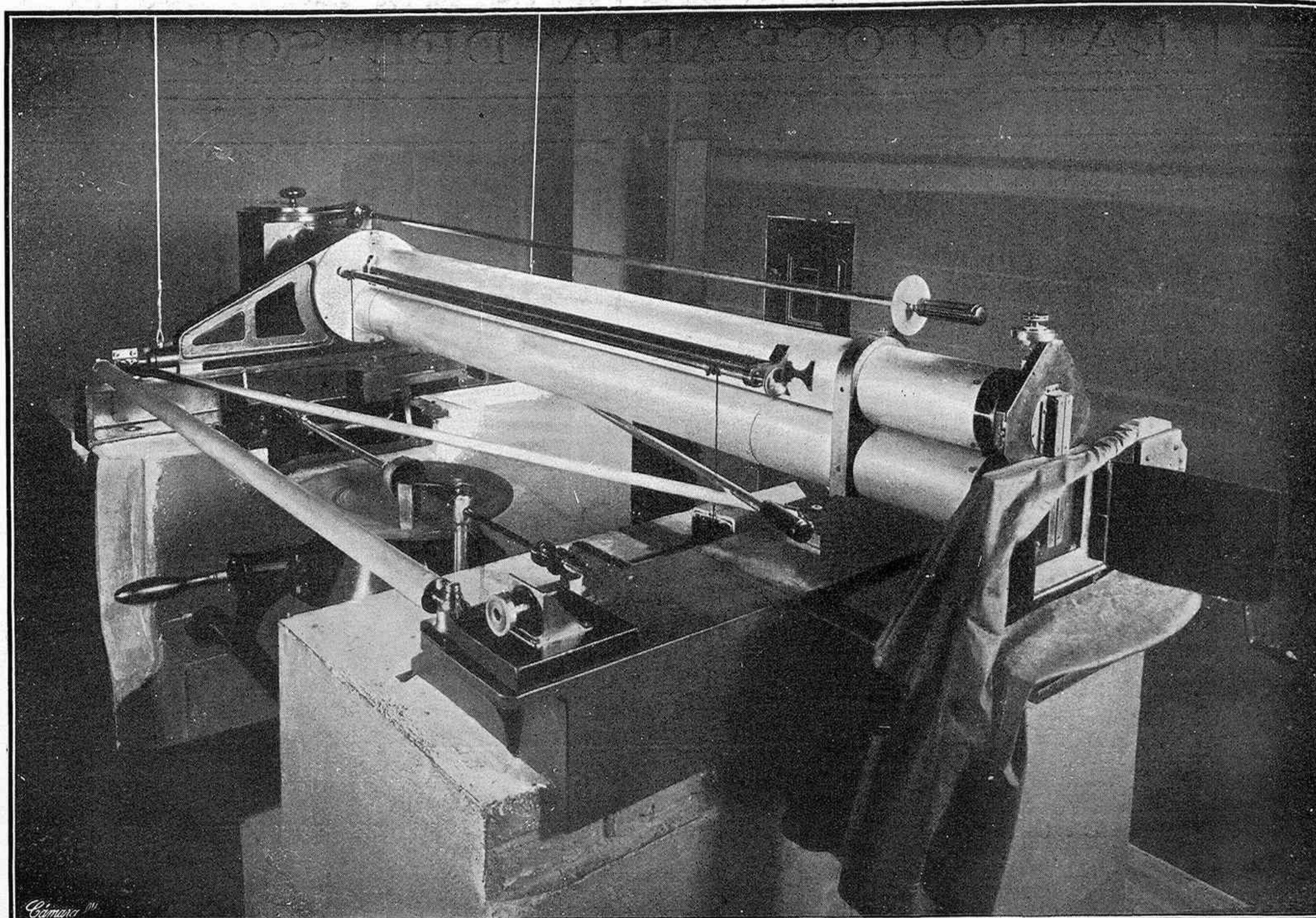
Espectroheliógrafo del Observatorio de Madrid, con el cual se descompone la luz del sol, se aísla de un cuerpo cualquiera y se obtienen imágenes solares con luz de calcio
