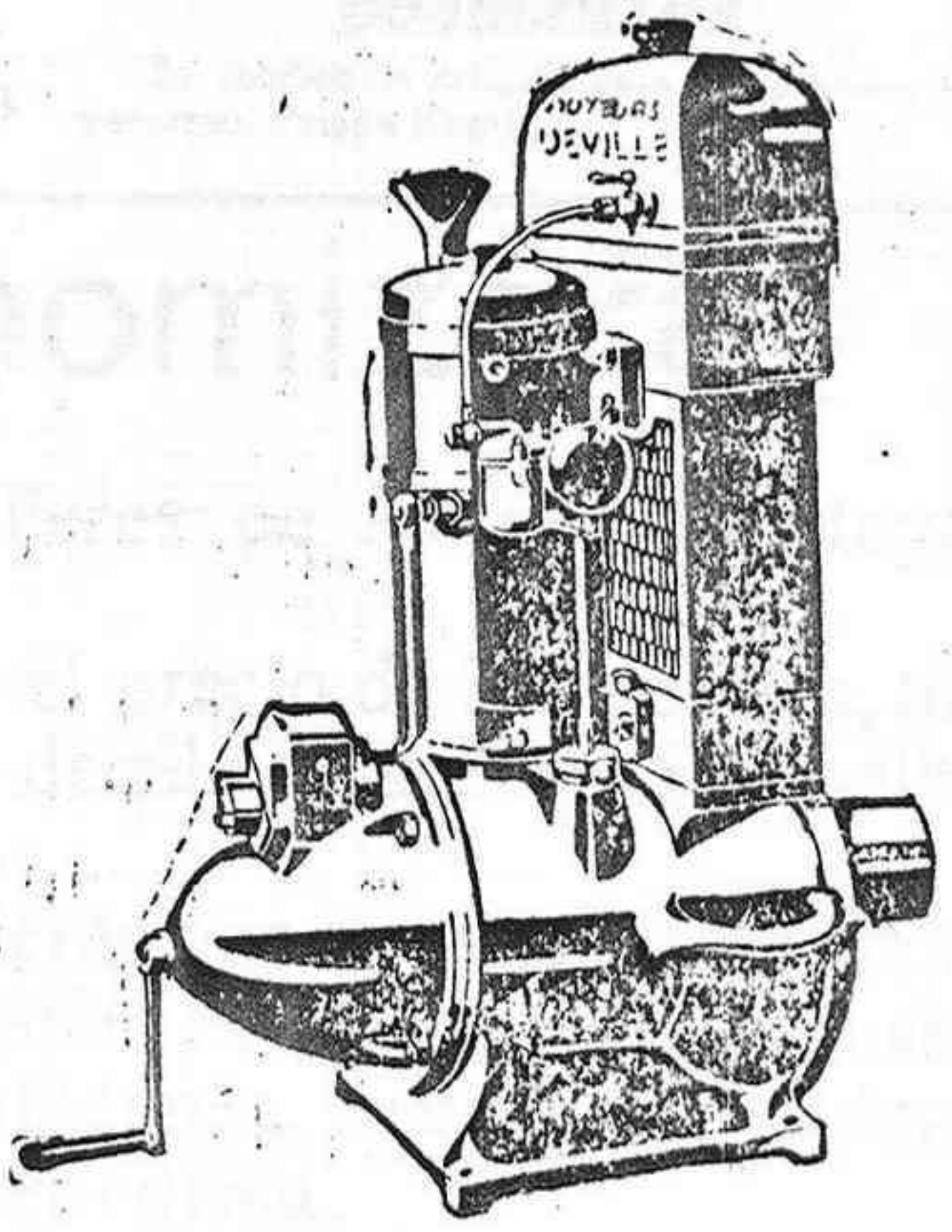
Motores a gasolina «DEVILLE» con radiador
