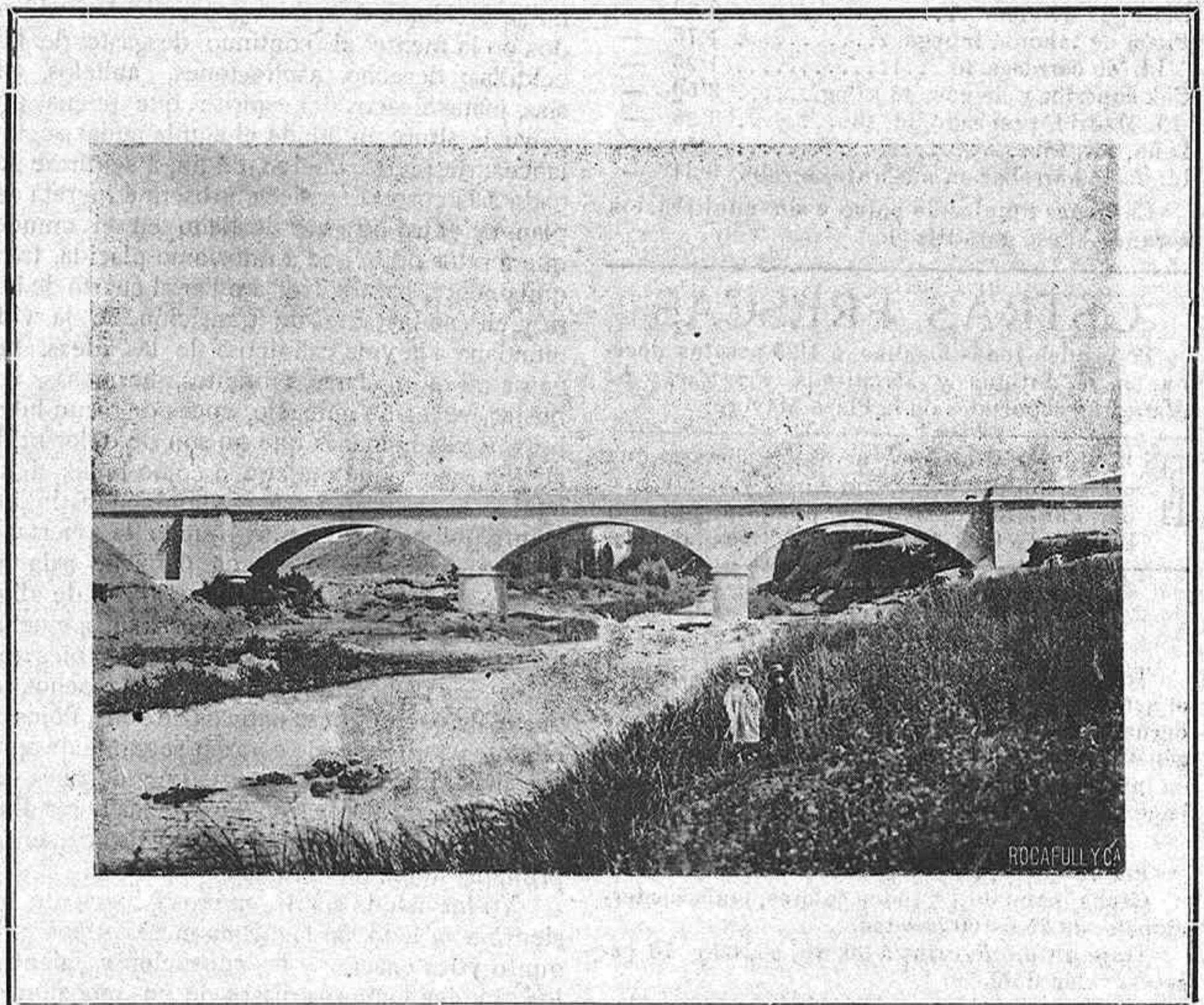
PUENTE SOBRE EL RÍO HENARES EN LA CARRETERA DE FONTANAR Á TÓRTOLA CUYA RECEPCIÓN OFICIAL SE VERIFICÓ EL DÍA 10 DEL CORRIENTE MES
