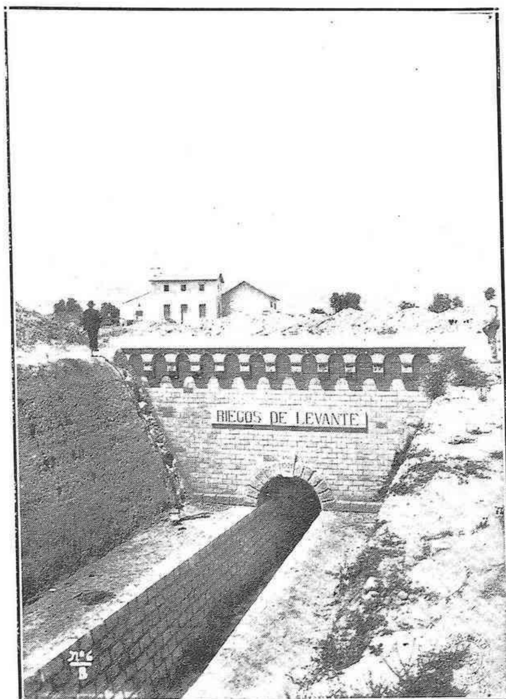
Canal general de conducción. Boquilla de entrada a la primera galería.
