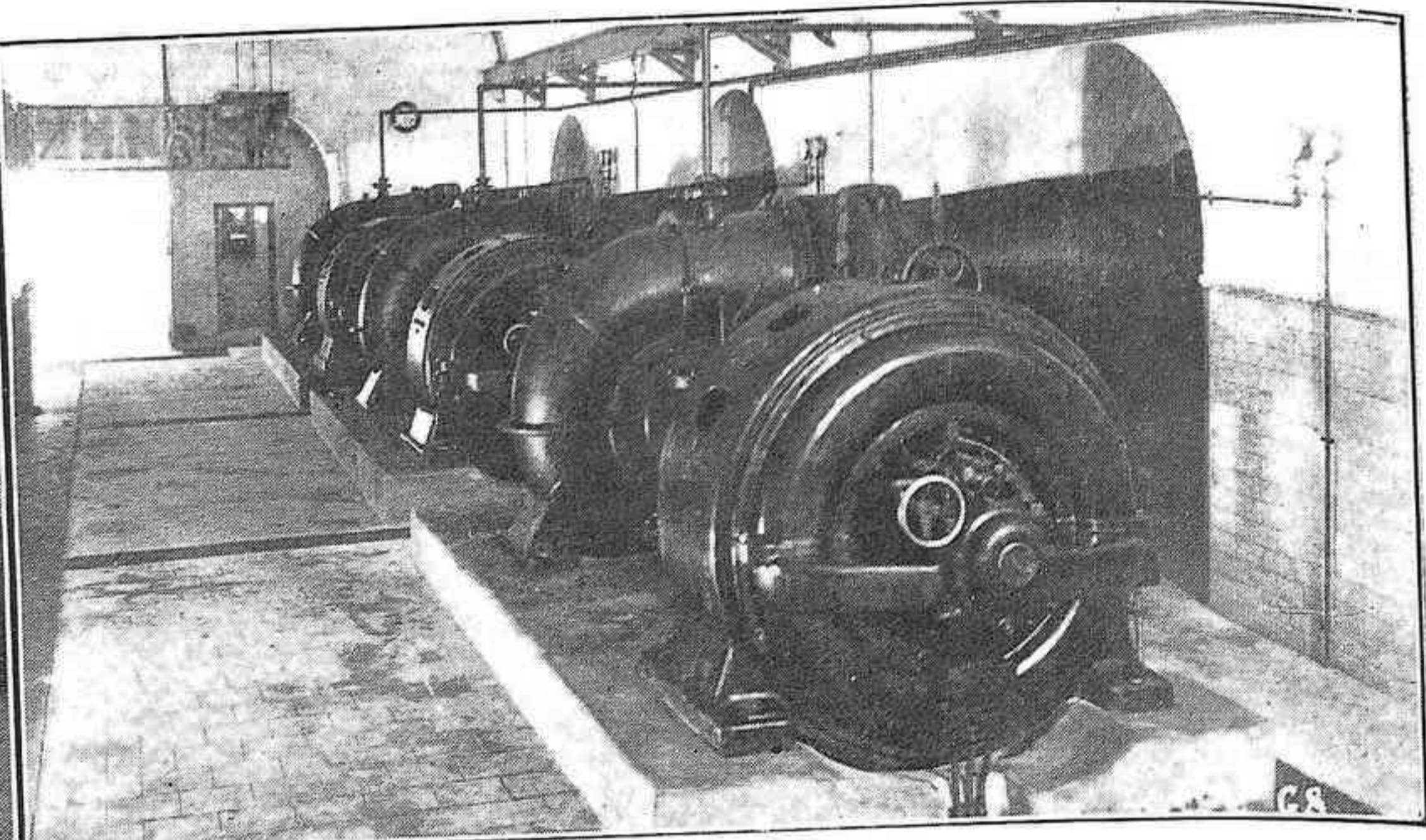
Tercera elevación subterránea. Tres bombas de 1.500 litros por segundo.
