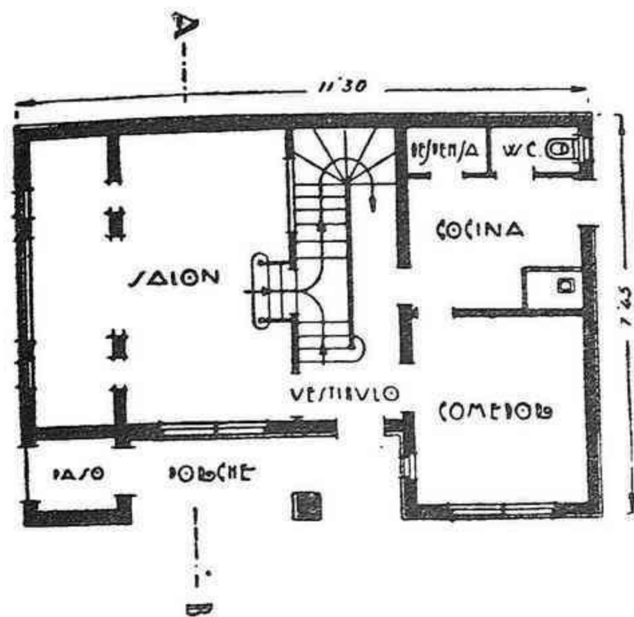
PLANTA BAJA
