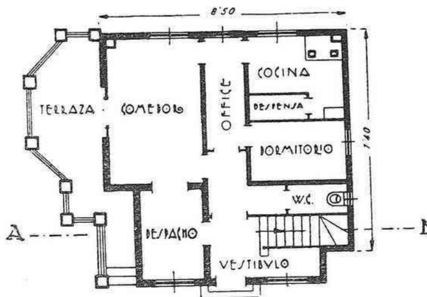
PLANTA BAJA
