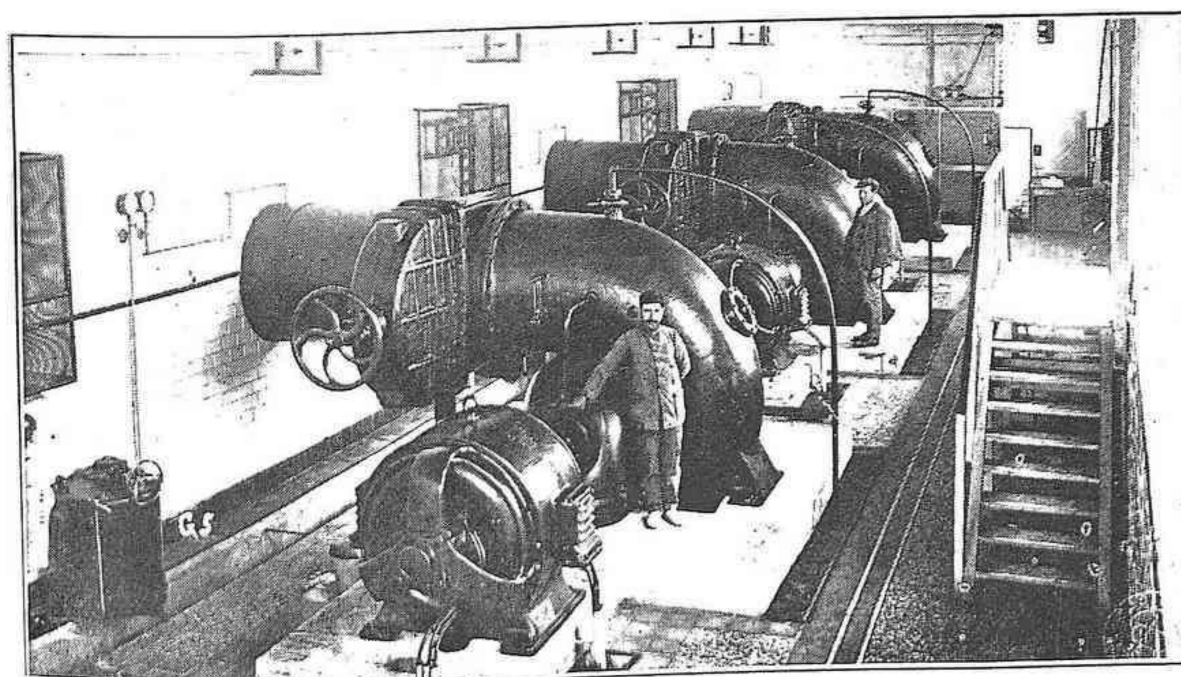
Interior de máquinas de la primera elevación.
