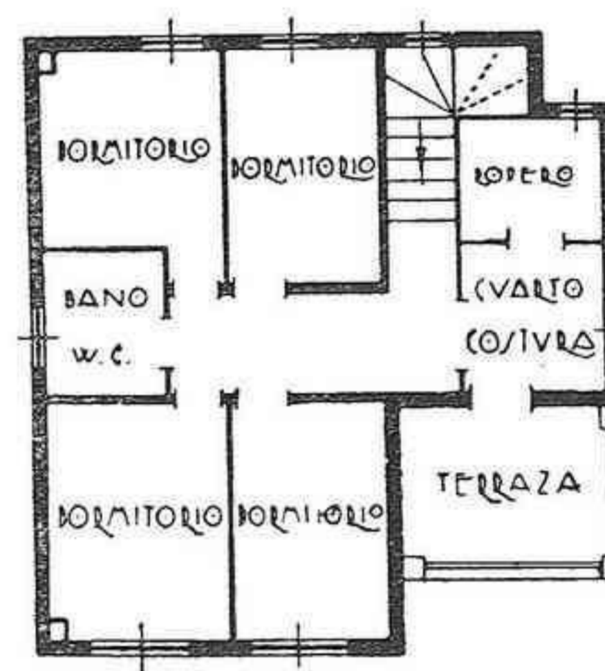
PLANTA PRINCIPAL
