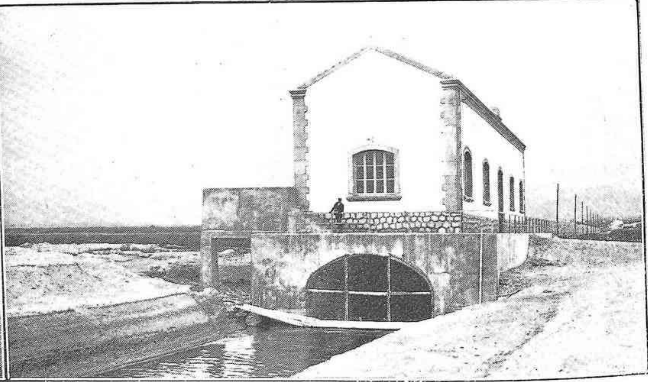
Casa de máquinas de la segunda elevación terminada.
