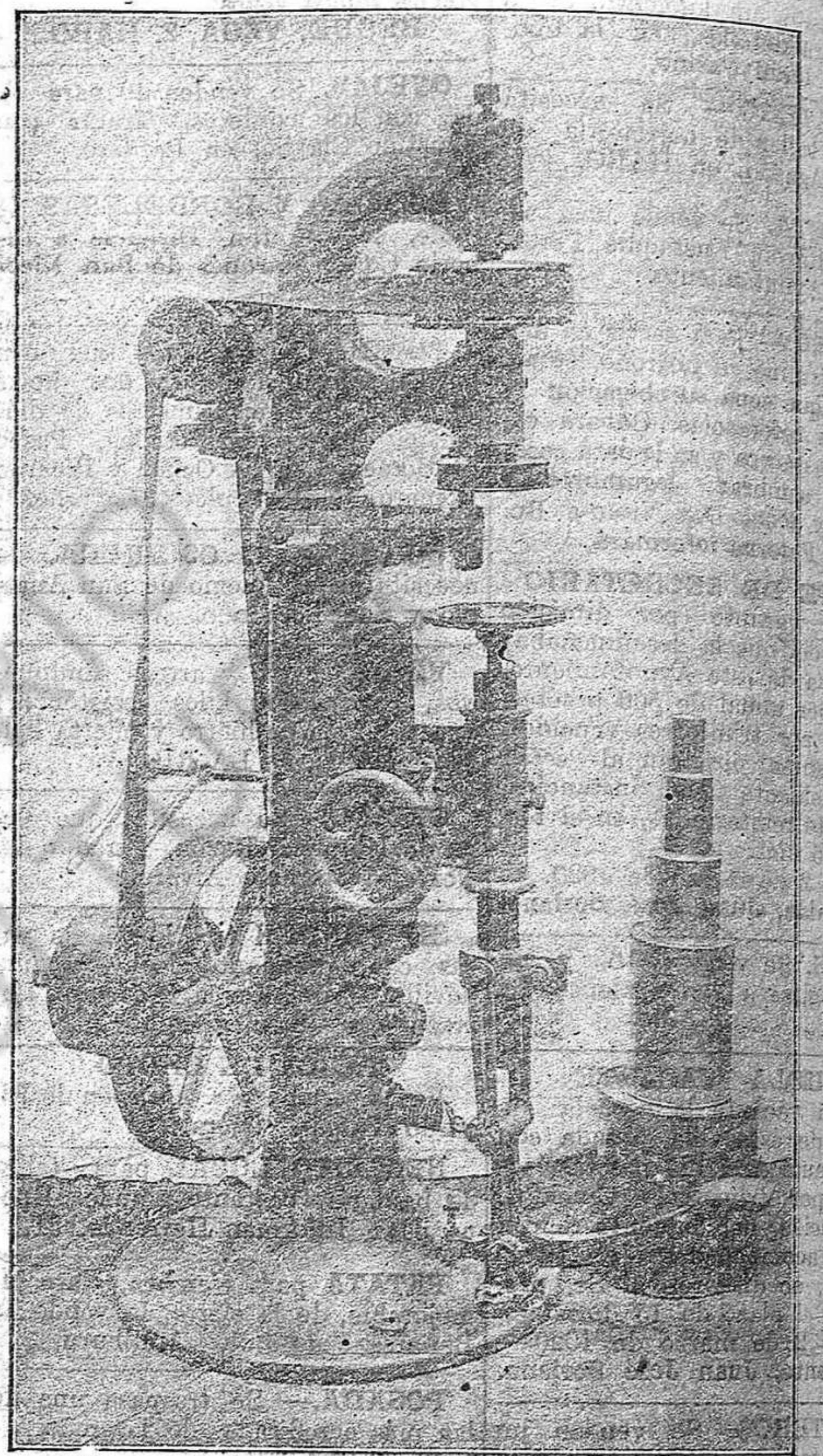
Máquina corrodora o encajadora para envases metálicos redondos. Pueden cerrarse toda clase de botellas redondas comprendidos entre 40 y 240 milímetros de diámetro. Esta máquina está construida con el mayor esmero; todos sus roces van encajados con bronce fosforoso. CONSTRUCTOR, FELIX PASCUAL OCHOA, CALLE JUAN LOBO, 8 Y 9, LOGROÑO.
