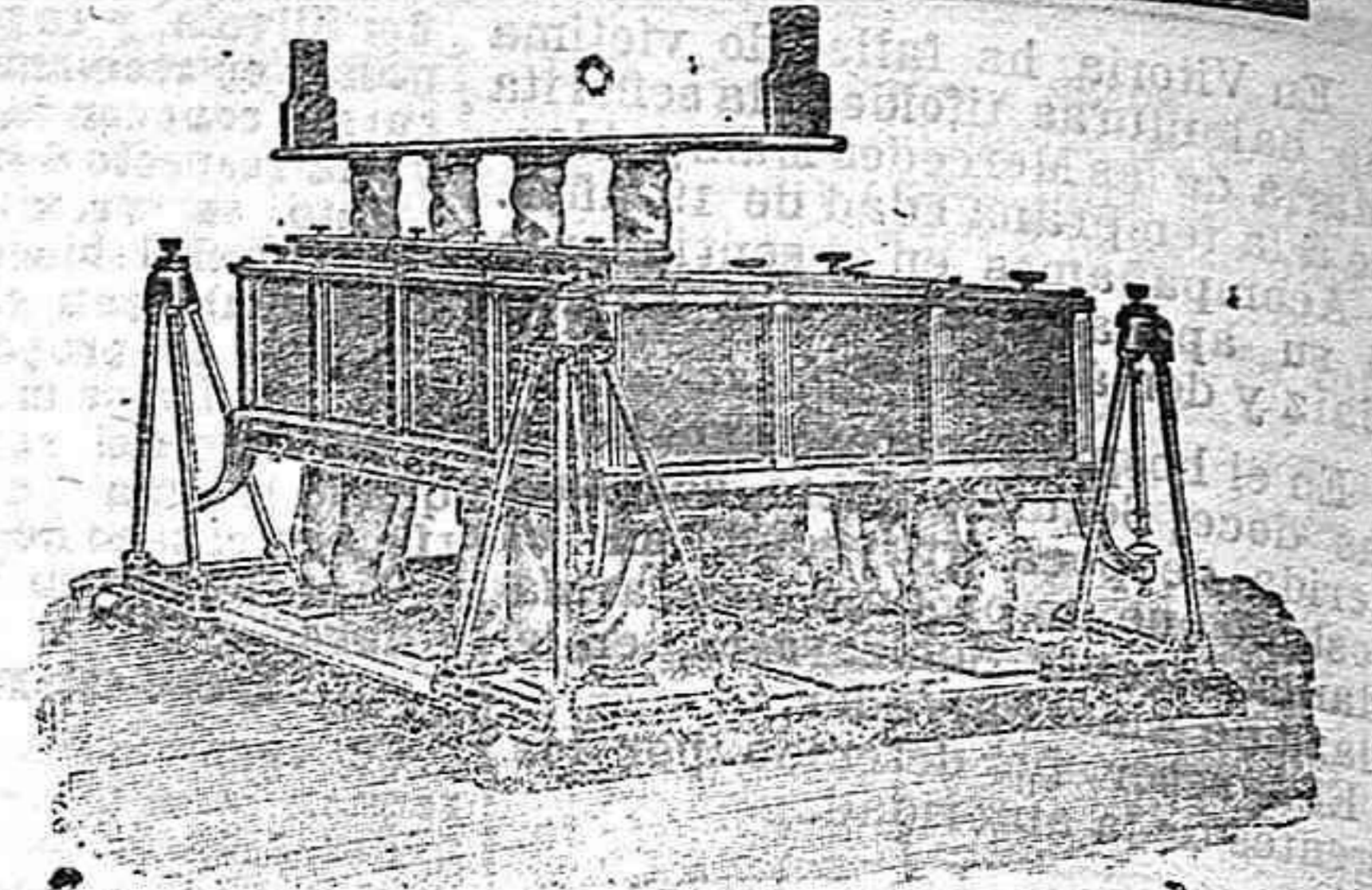
Plansichter DAVERIO, construcción 1902
