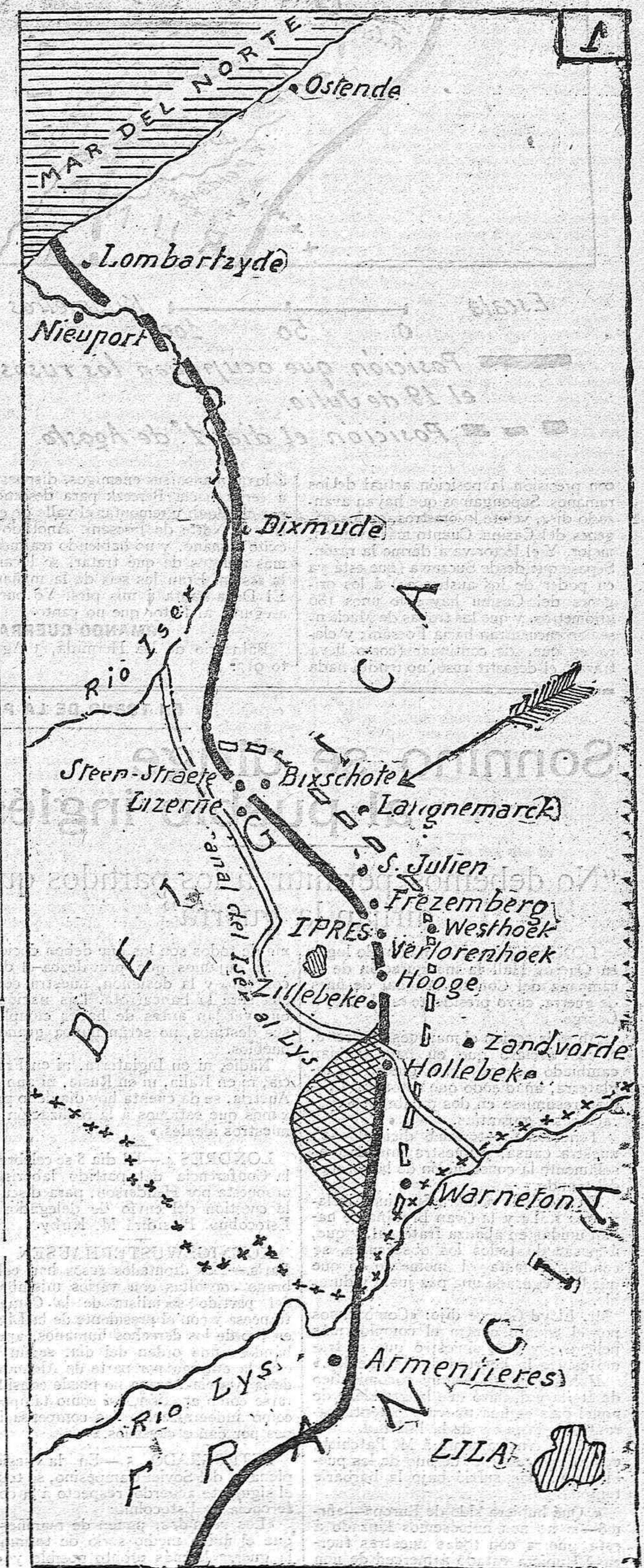
Escala por Kilometros 0 2 4 6 8 10 Frontera franco-belga. Canal del Iser al Lys. Posición que ocupaban los alemanes el día 31 de Julio. Posición que ocupaban los alemanes el 1.º de Agosto.
