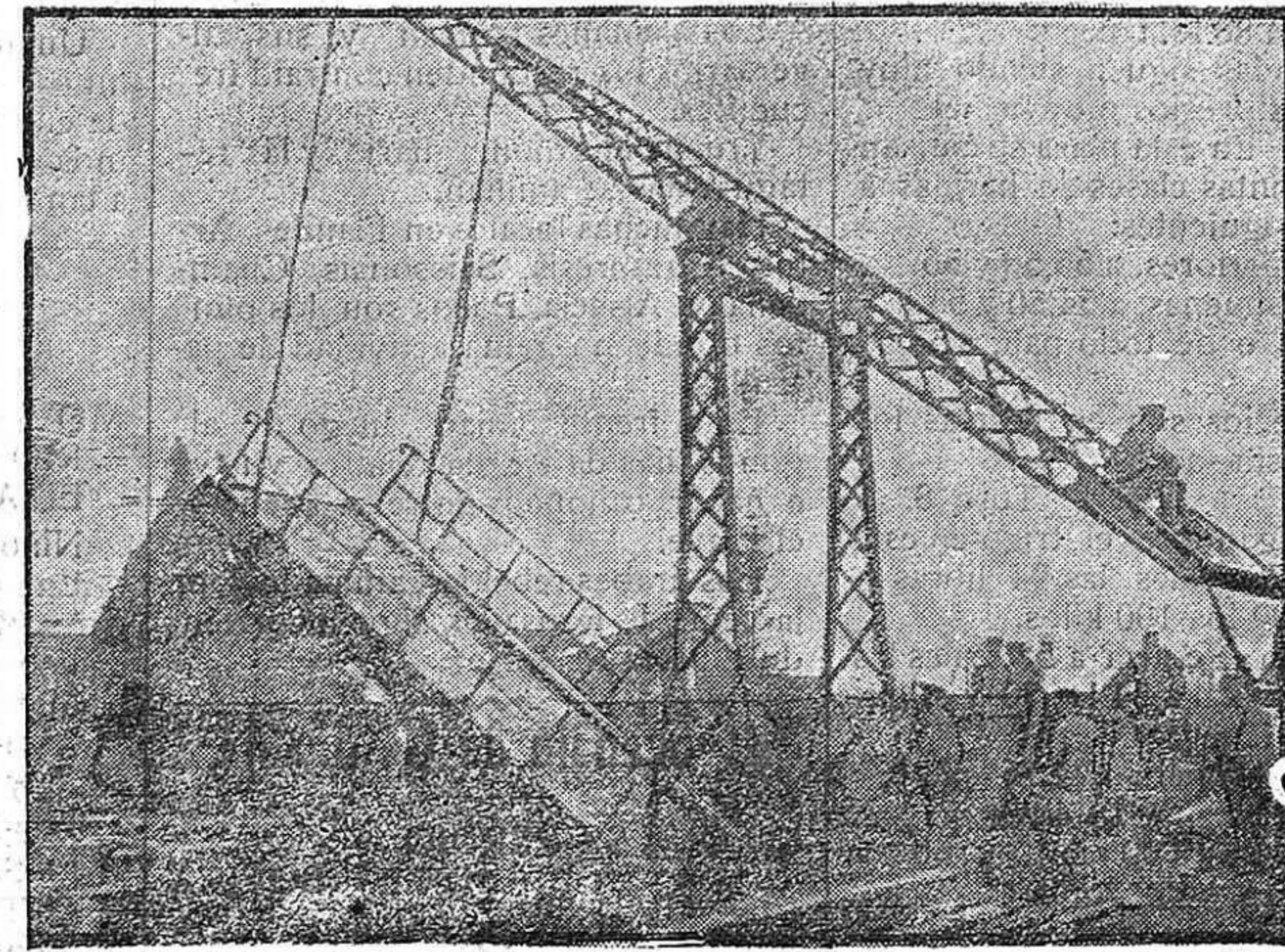
DE LA GUERRA.—Construcción de un puente sobre el canal del Somme.
