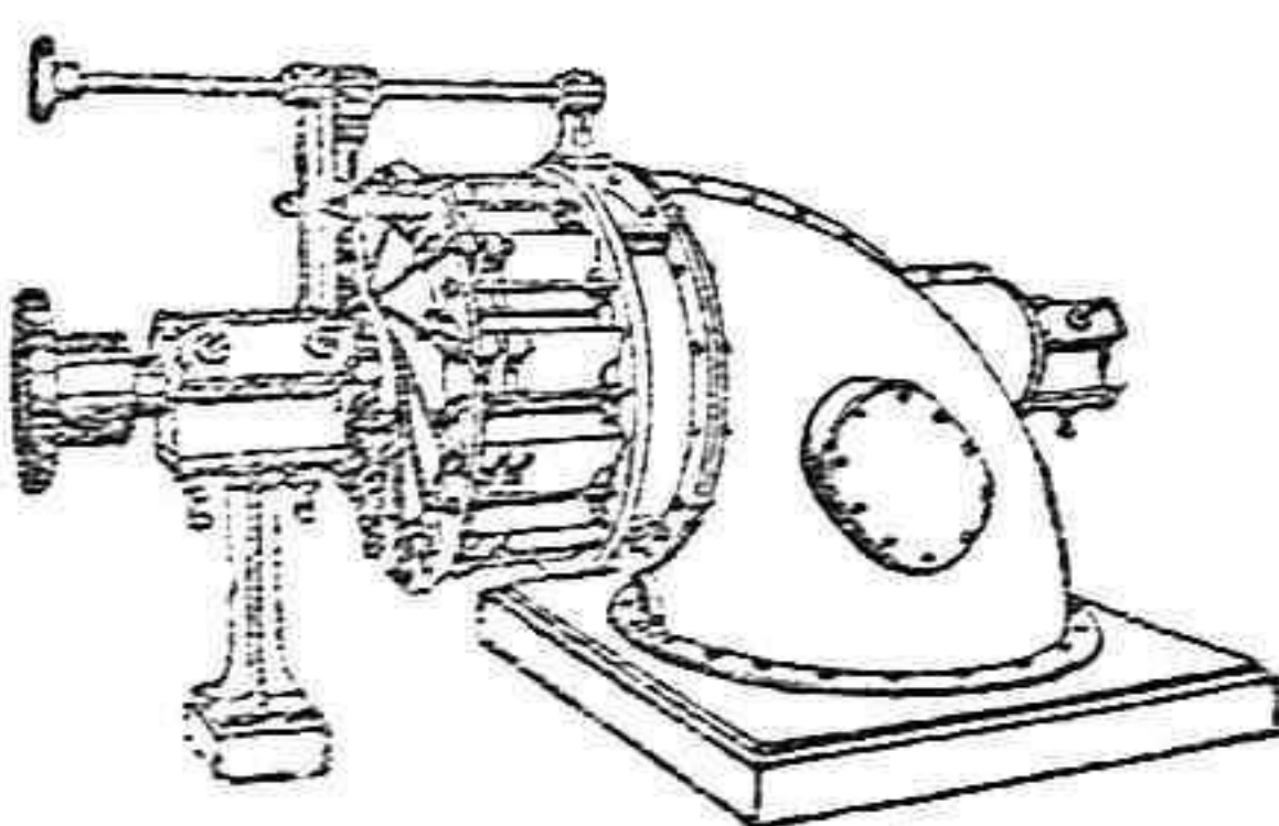
Turbina horizontal (Samson)
