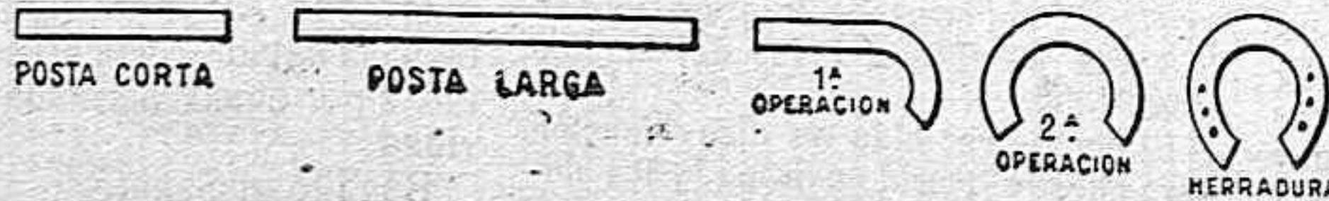
RECORTES Y PLETINAS PARA FABRICACIÓN DE HERRADURAS.
