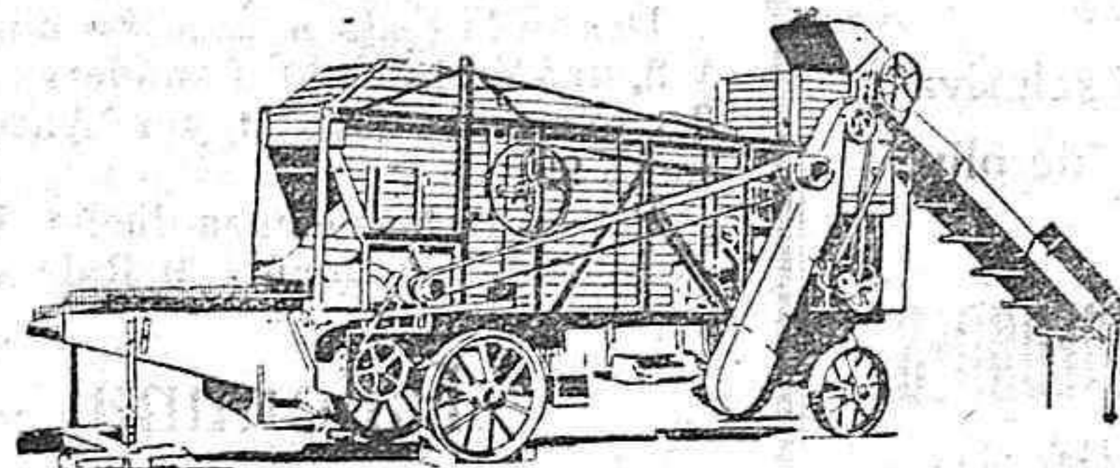
Trilladora «Triunfo Grande» con elevador de mies. Rendimiento diario de 150 a 200 fanegas de trigo, según granazón.
