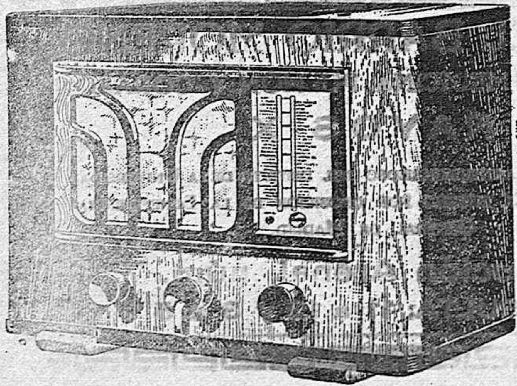
510 A. 6 válvulas. Corriente alterna, todos los voltajes Escala con nombre de emisores. Selectividad extraordinaria. Ptas. 555 510 U. Iguales características, para todas las corrientes. Ptas. 565
