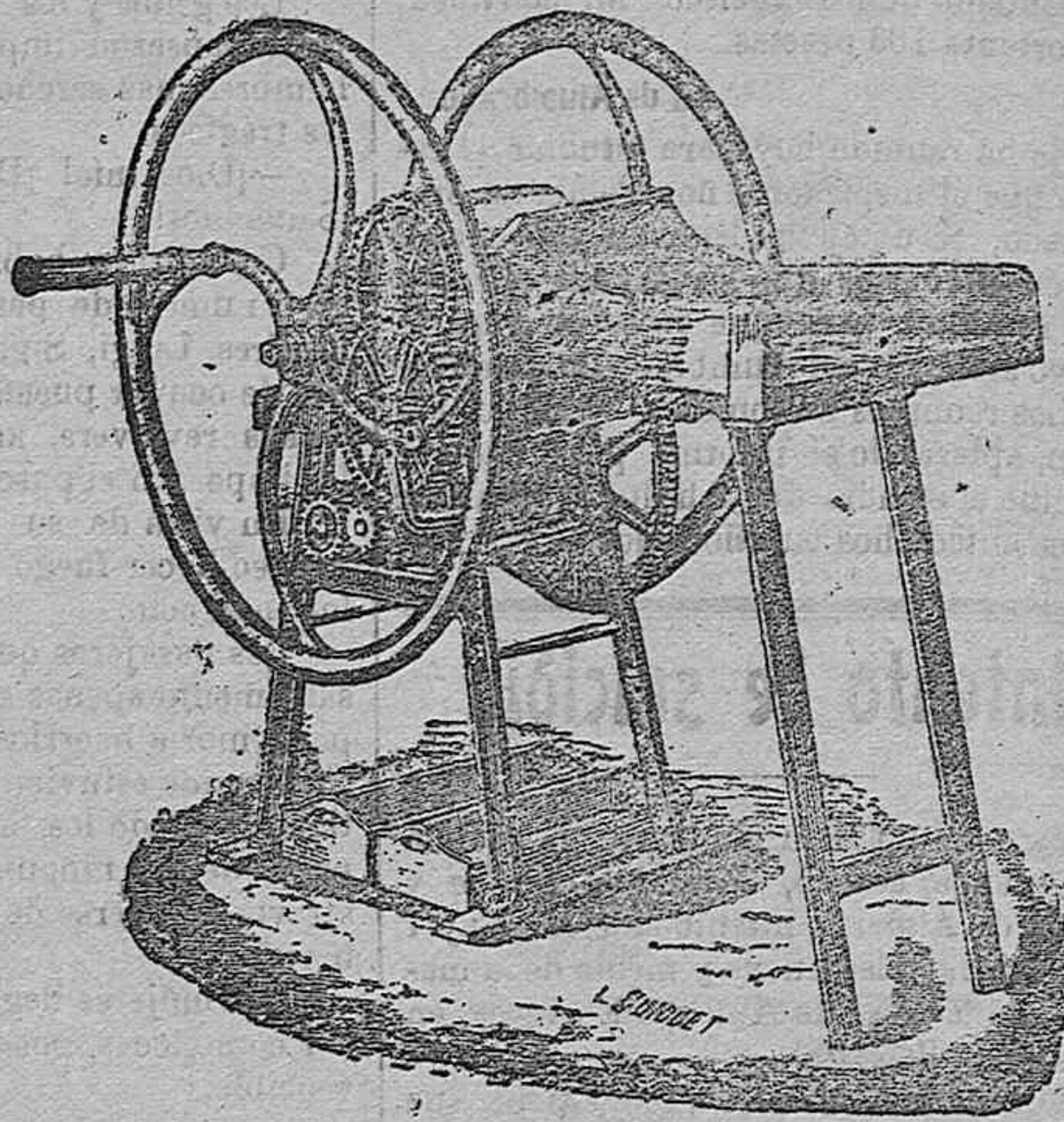
Machacadora de auлага s r mientos
