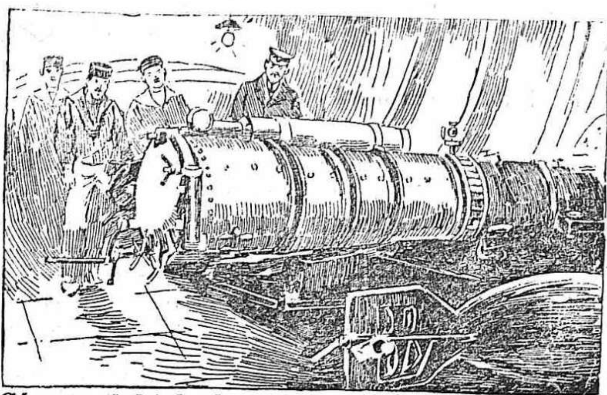
Cámara del tubo lanza-torpedos del submarino «El Volta»
