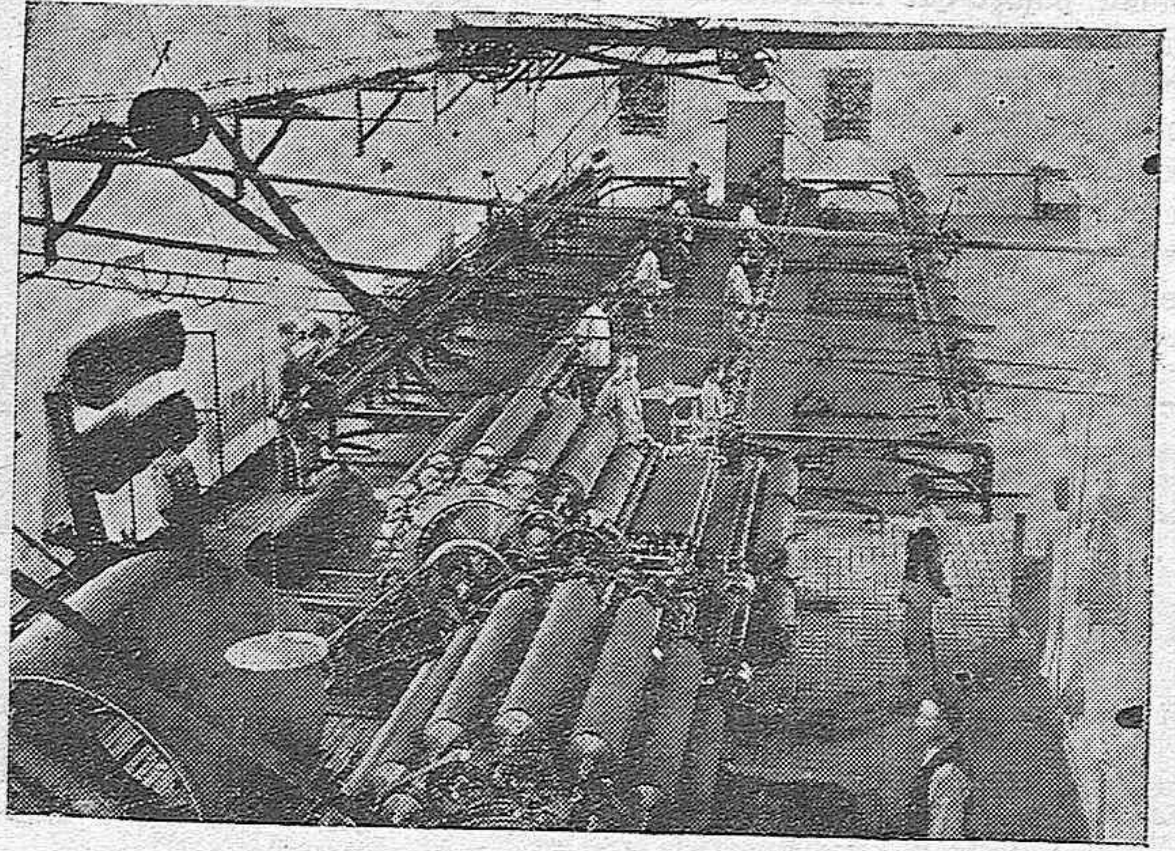
Vista de la sala de máquinas de hilados de la gran fábrica de tejidos de don Rafael Muñoz Cabrera .
