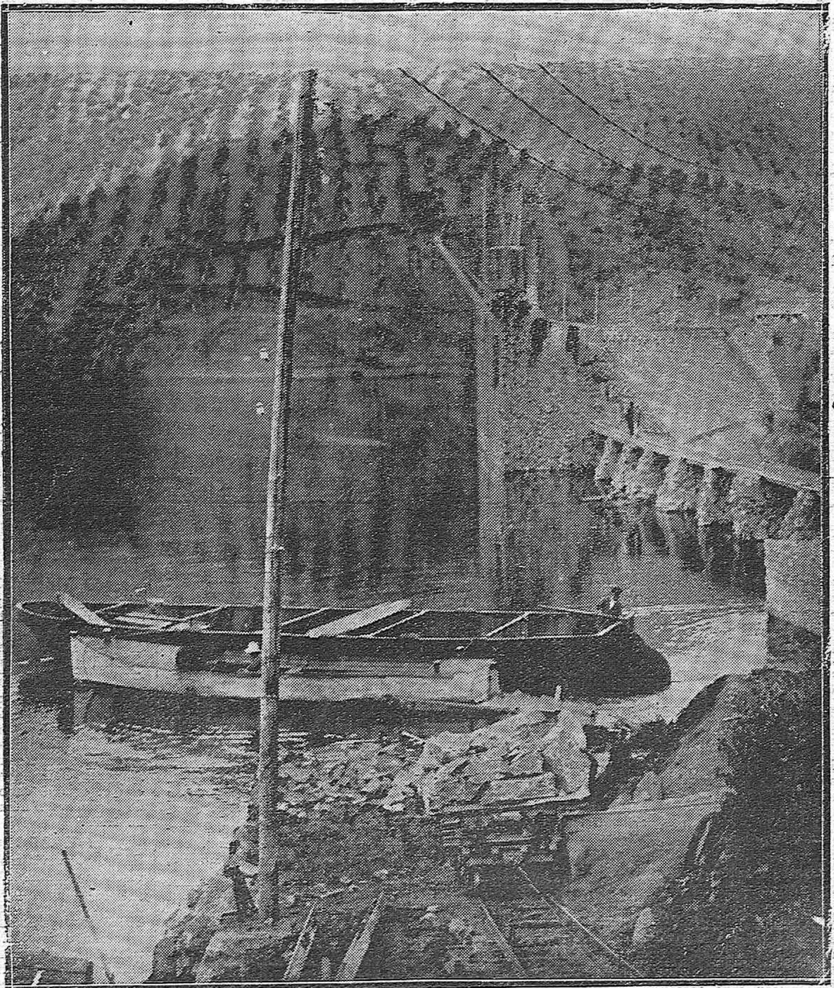
EL PANTANO DEL GUADALMELLATO.—ESTADO ACTUAL DE LAS OBRAS DEL IMPORTANTE PANTANO.
