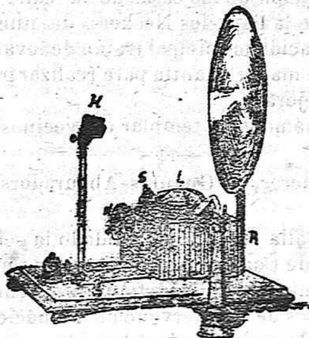
Aparato receptor del teléfono de acetileno
