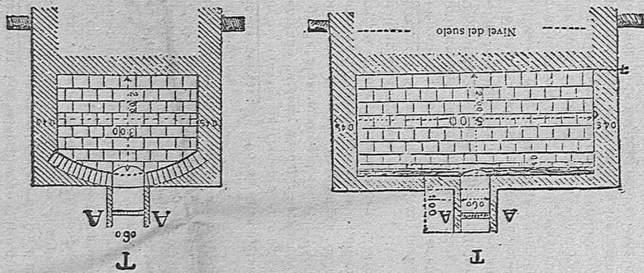
Croquis de un Depósito con revestimiento de BALDOSINES DE VIDRIO construido sobre el nivel del suelo
