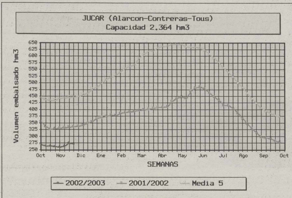
Análisis de la reserva hídrica en el sistema Alarcón-Contreras-Tous.
