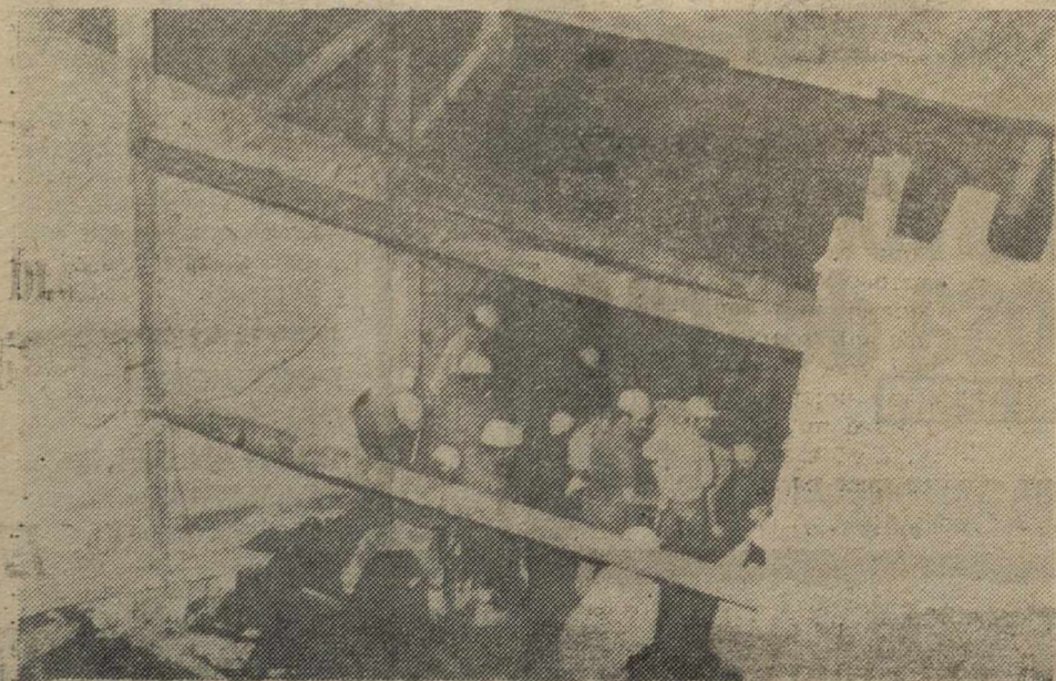
BARCELONA.—Tres obreros muertos y dos heridos, al quedar atrapados por el hundimiento de parte de la bóveda de las obras en construcción del Metro de la Avenida del Marqués del Duero, esquina a Ricart. En la foto, una vista parcial de la bóveda derruida.—(Telefoto CIFRA GRAFICA)
