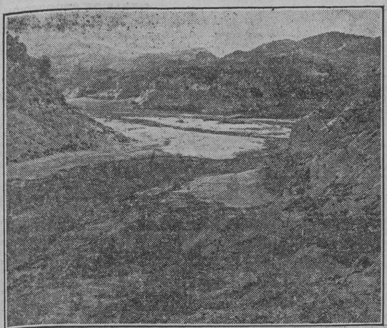
Magnífica perspectiva de la taza del pantano de Tibi, que embalsa cerca de cuatro millones de metros cúbicos de agua.
