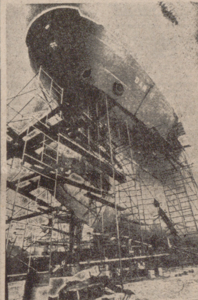
El «Darro», de 3.400 toneladas, es el mayor buque construido hasta ahora en astilleros santanderinos. Tiene 111,50 metros de eslora y 15,75 de manga. Será botado en abril. (Foto Cifra Gráfica)
