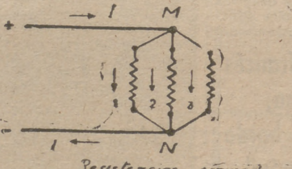
Resistencias derivadas conexión en paralelo
