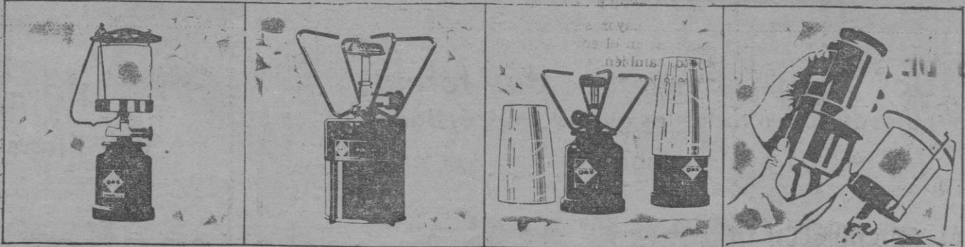
LUMOGAS "C" Altura: 30 cms. Diám.: 10 cms. MINIGAS "S" Altura: 20 cms. Diám.: 9 cms. MINIGAS "L" Altura: 24 cms. Diám.: 10 cms. Peso: 810 grs. Consumo: 20 a 30 grs. por h. Peso: 415 grs. Consumo: 50 grs. por hora. Peso: 580 grs. Consumo: 50 grs. por hora.
